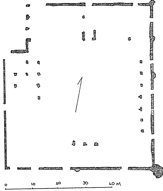
Şek. 9-Hurmuzfarra Kervansarayı. Plan (Pugaçenkova'nın planına göre).
