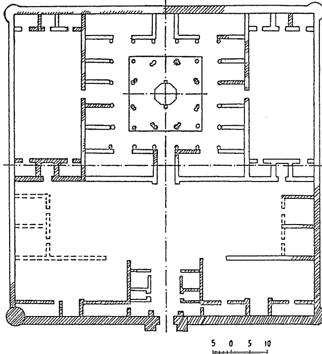
Şek. 14-Ribat-ı Melik. II. İnşa Evresi Planı (N. B. Nemtseva).
