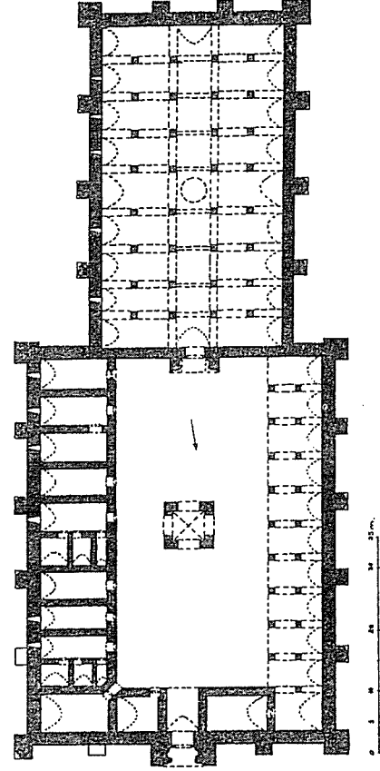
Şek. 21- Sultan Hanı (Konya-Aksaray). Plan (K. Erdmann).
