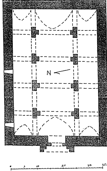
Şek. 24-Eğret Hanı. Plan (K. Erdmann).
