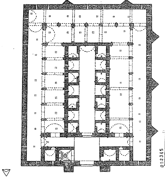
Şek. 27-Alara Hanı. Plan (A. Y. Tükel).
