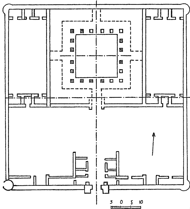
Şek. 13-Ribat-ı Melik. I. İnşa Evresi Planı (N. B. Nemtseva).
