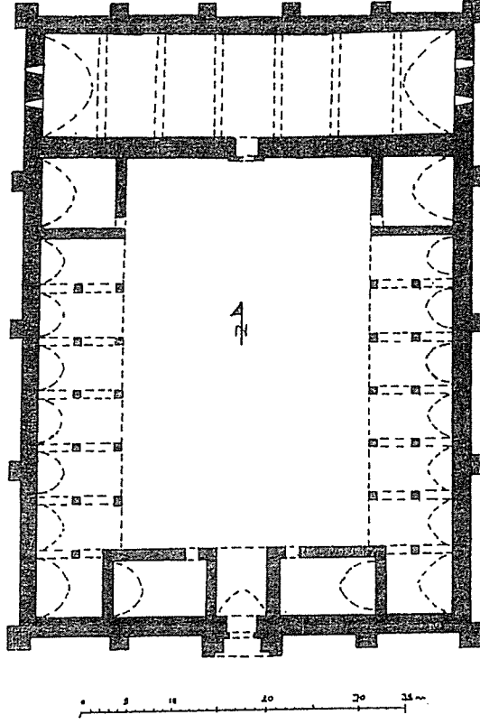
Şek. 23-Kırkgöz Hanı. Plan (K. Erdmann).
