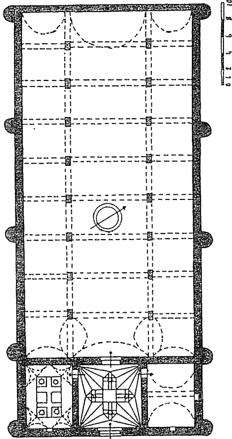
Şek. 25-İğdir Hanı. Plan (R. H. Ünal).
