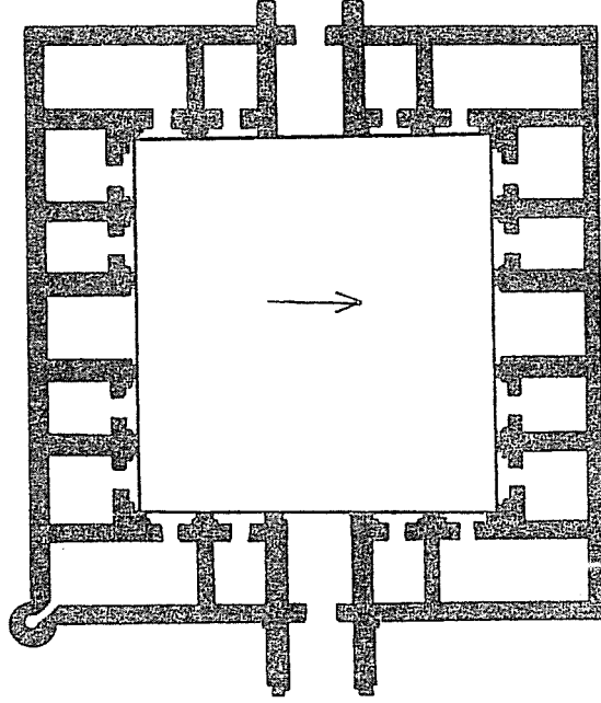
Şek. 1- Ode-Merguen Kervansarayı. Plan (G. A. Pugaçenkova).
