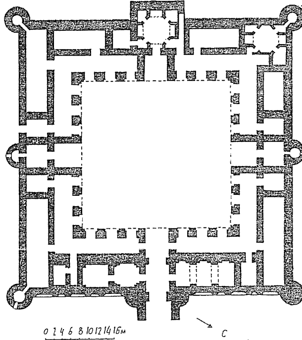
Şek. 4-Daya Hatun Kervansarayı. Plan (G. A. Pugaçenkova).
