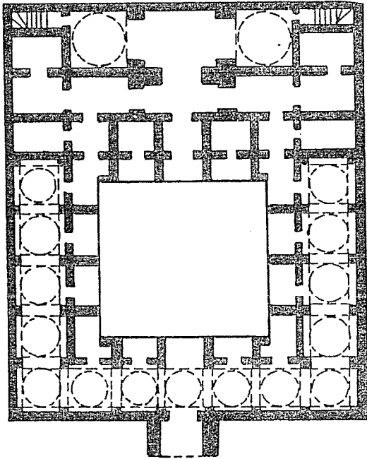
Şek. 6-El Asker Kervansarayı. Plan (G. A. Pugaçenkova).
