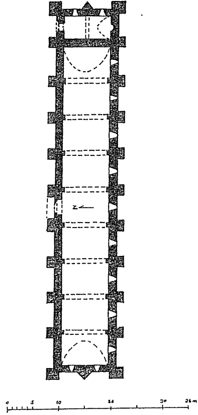
Şek. 26-Şarapsa Hanı. Plan (K. Erdmann).
