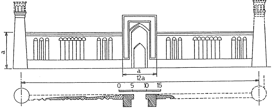
Şek. 12-Ribat-ı Melik. Cephe Çizimi (N. B. Nemtseva).
