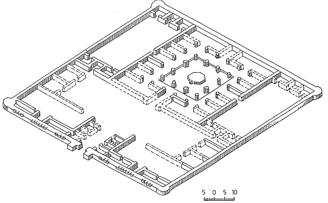
Şek. 15-Ribat-ı Melik. Aksonometrik Çizimi (N. B. Nemtseva).
