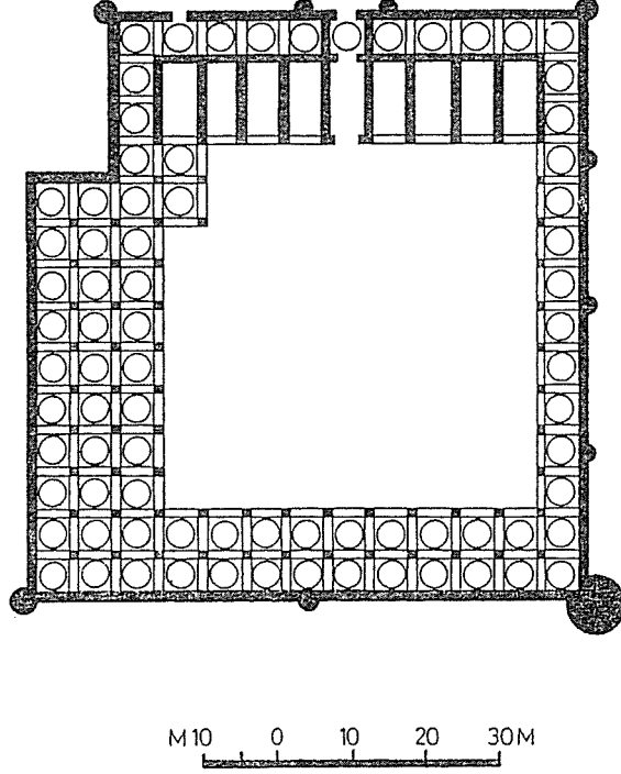
Şek. 8-Hurmuzfarra Kervansarayı. Plan (M. E. Masson).
