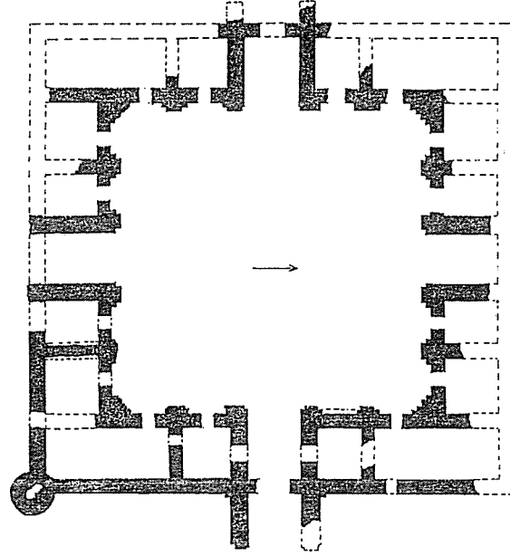
Şek. 2- Ode-Merguen Kervansarayı. Plan (Pugaçenkova'nın planına göre)
