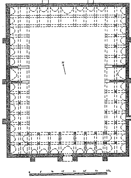
Şek. 22-Evdir Hanı. Plan (K. Erdmann).
