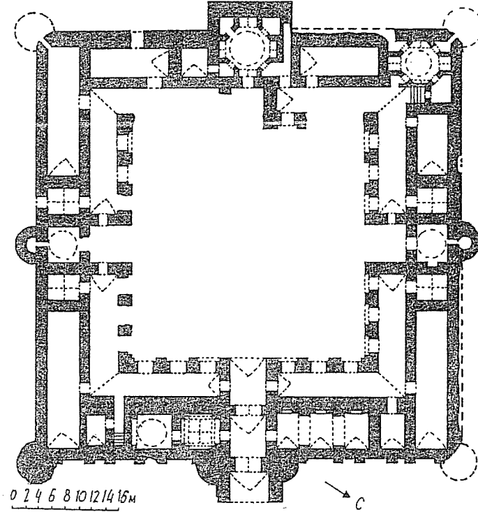
Şek. 5-Đaya Hatun Kervansarayı. Plan (Pugaçenkova'nın planına eklemelerle).
