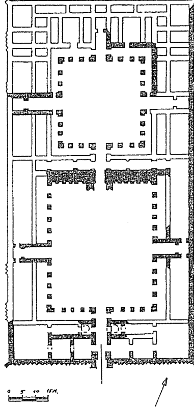
Şek. 11-Akçakale Kervansarayı. Plan (G. A. Pugaçenkova).
