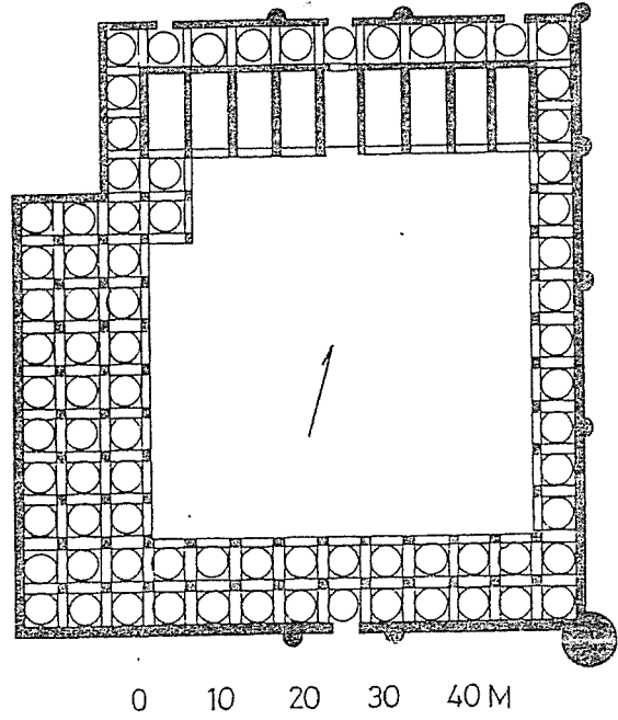
Şek. 7-Hurmuzfarra Kervansarayı. Plan (G. A. Pugaçenkova).
