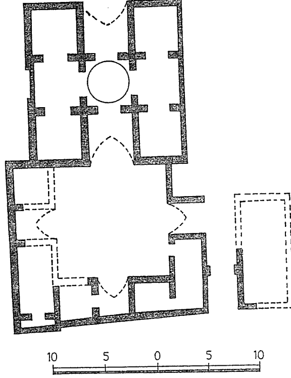
Şek. 19-Kurtlutepe Kervansarayı. Plan (M. E. Masson).
