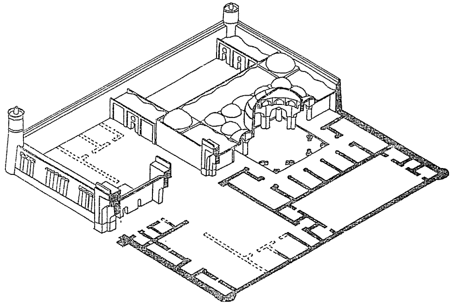
Şek. 16-Ribat-ı Melik. Aksonometrik Çizimi (N. B. Nemtseva).
