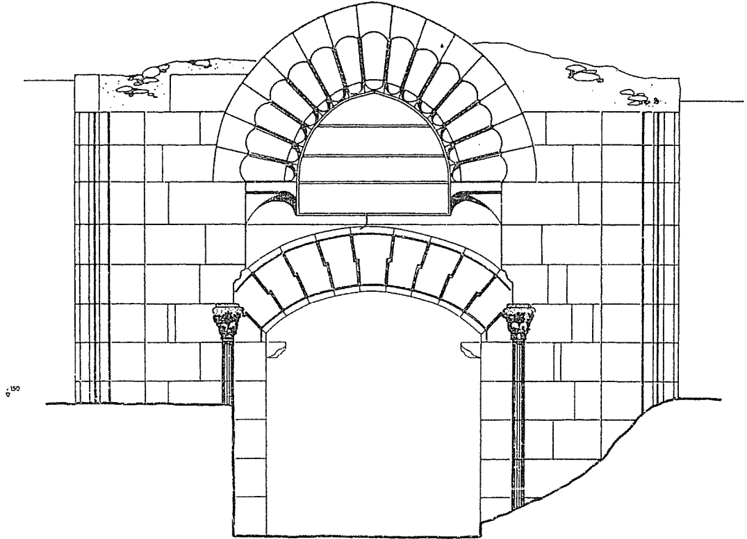
Şek. 6- İncir Hanı. Ahır taçkapısı (Rölöve ve çizim E. Gültekin).
