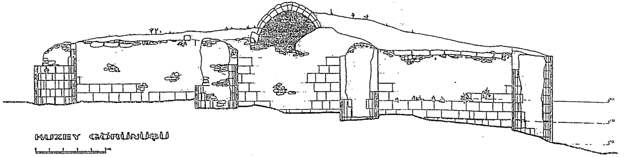
Şek. 4- İncir Hanı. Ahırın kuzey cephesi (Rölöve ve çizim E. Gültekin).
