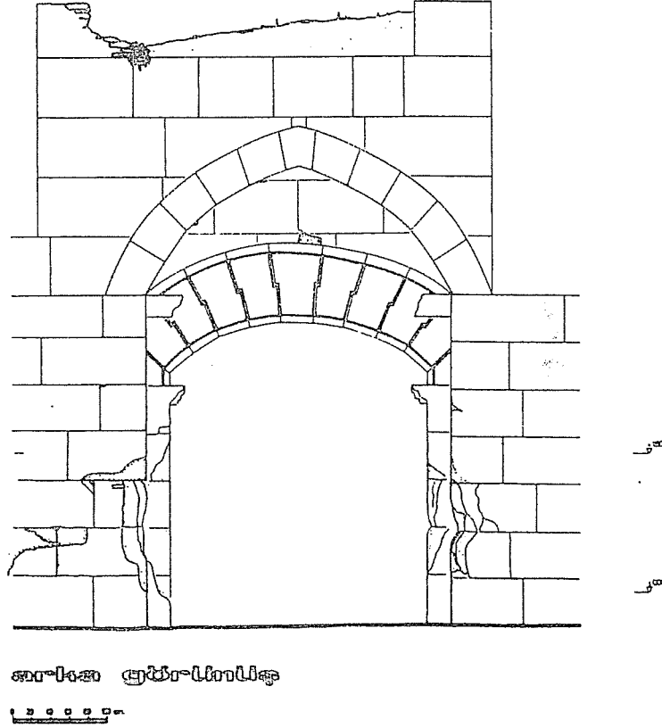
Şek. 9- İncir Hanı. Ahır girişinin içten görünüşü(Rölöve ve çizim E. Gültekin).
