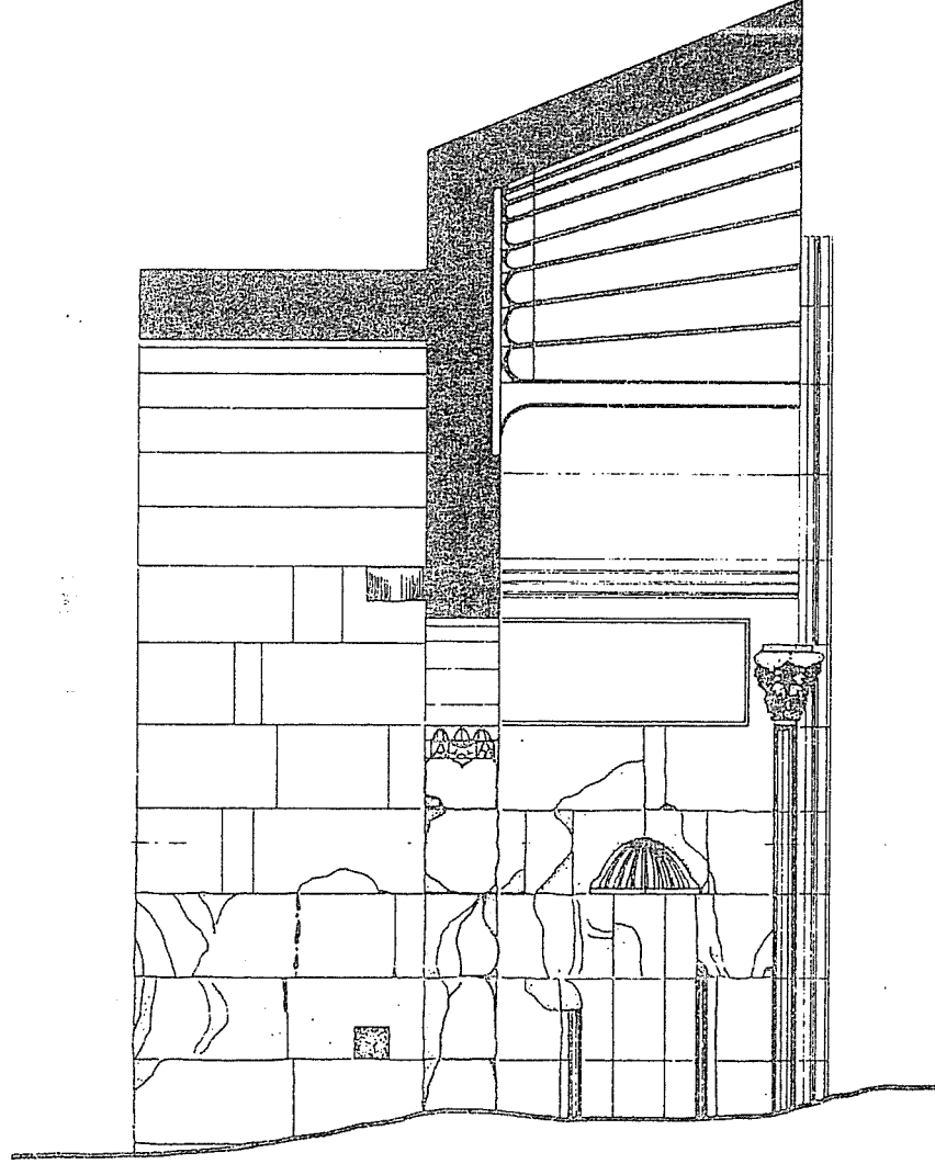
A-A kesiti
