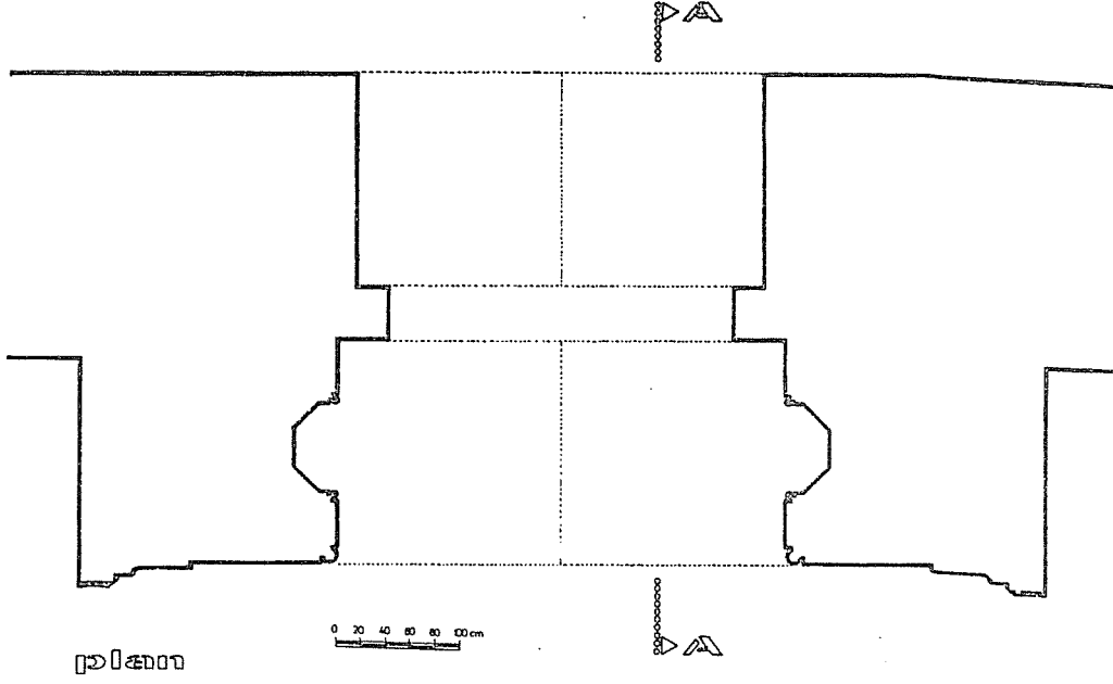
Şek. 7- İncir Hanı. Ahır taçkapısı planı (Rölöve ve çizim E. Gültekin).
