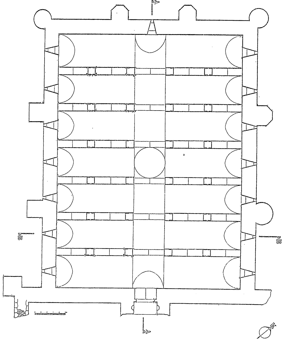
Şek. 1- İncir Hanı. Ahırın planı (Rölöve ve çizim E. Gültekin).
