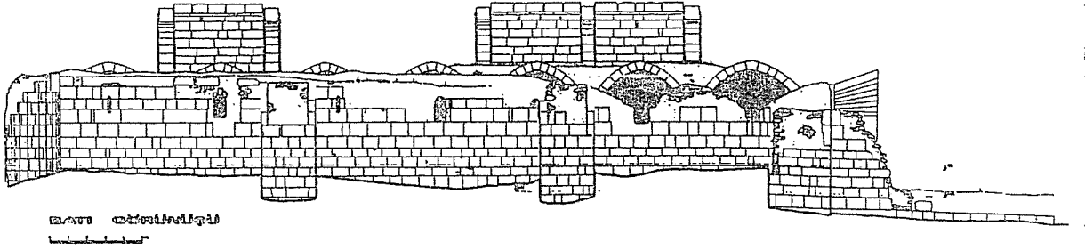
Şek. 3- İncir Hanı. Ahırın batı cephesi (Rölöve ve çizim E. Gültekin).
