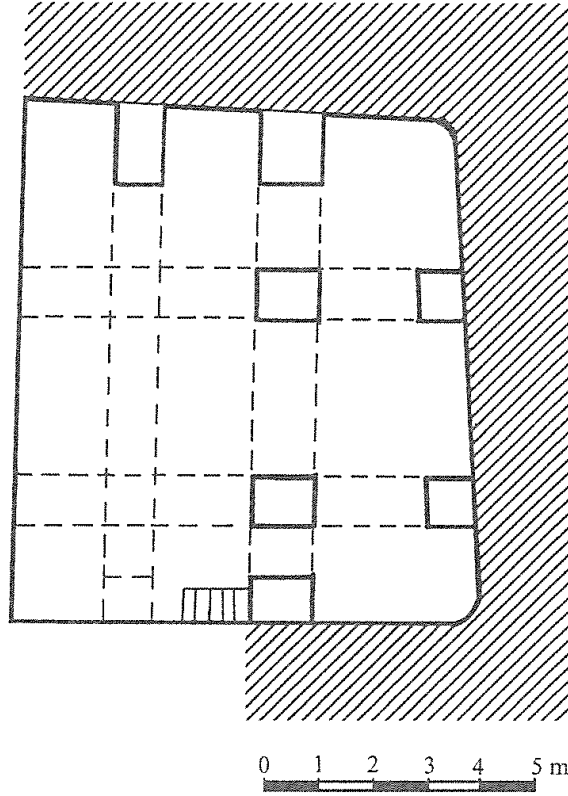
Plan 1- Oxia Manastırı, II. nolu sarnıç planı (Çiz: Mim. Haldun Özyurt-1997).
