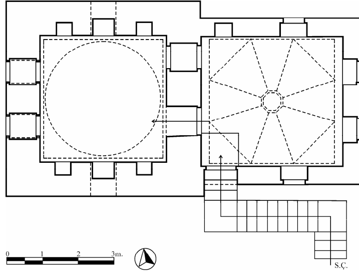
Şek.2- Gebze, Çoban Mustafa Paşa Külliyesi Kütüphanesi, planı.
