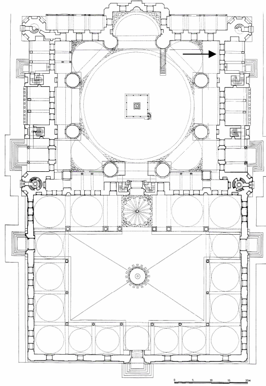
Şek.3- Edirne, Selimiye Camii, planı (Ç. Birkan'dan).
