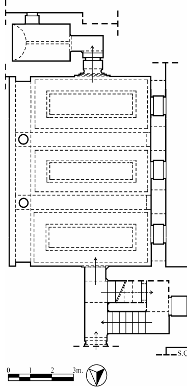
Şek.4- Edirne, Selimiye Camii Kütüphanesi, planı.
