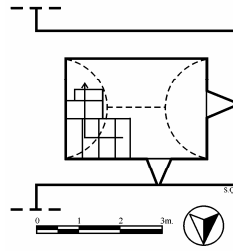
Şek.5- Edirne, Selimiye Camii Kütüphanesi, merdiven sahanlığı üst kat planı.
