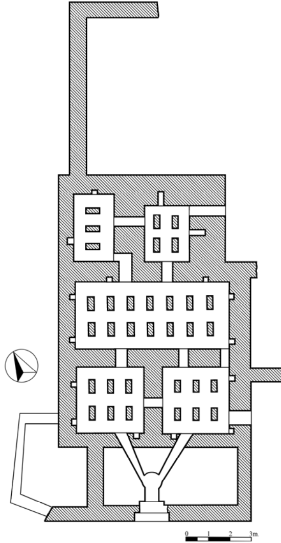
Şek.3-Seymenlik Zaviyesi Hamamı. Cehennemlik Katı Planı. (Rölöve ve Çizim Ş.Çakmak).
