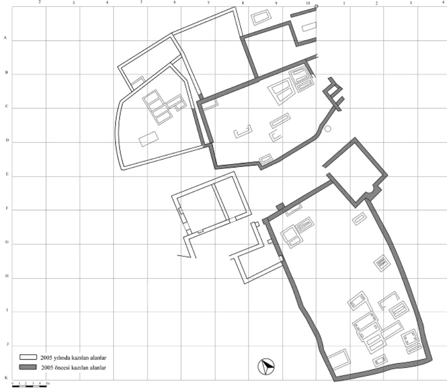
Şek.4- Mentеше Mezarlığı Vaziyet Planı (Rölöve ve Çizim E.Daş)
