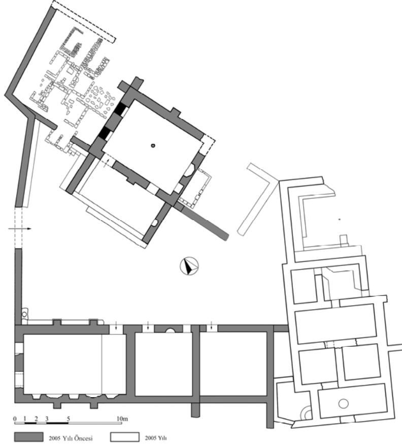
Şek.1- Seymenlik Zaviyesi vaziyet planı. (Rölöve ve Çizim Ş.Çakmak)
