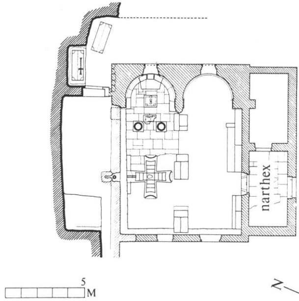
Çiz. 2a-b -Alahan Manastırı vaftiz binasının planı (M. Gough, An Early Christian Monastery in Southern Turkey , 1985, a- Fig. 62; b- Fig. 65.)
