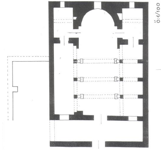
Çiz. 6- Seyranlık kilisesi planı (A. Aydın, “Mersin-Silifke, Seyranlık Köyü Geç Antik-Bizans Dönemi Mimarisi”, 21. AST, C. I, 2004, Çiz. 4.)
