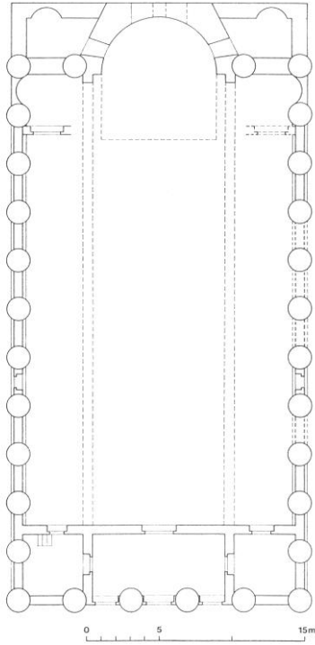
Çiz. 8- Uzuncaburç, Tapınak kilisesi planı (F. Hild- H. Hellenkemper-G. Hellenkemper-Salies, "Kommagene-Kilikien-Isaurien", RBK IV, 1990, 242 vd. Abb. 25)
