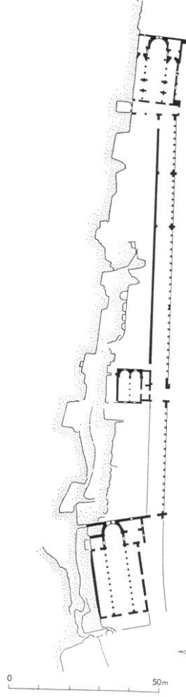
Çiz. 1 - Alahan Manastırı genel planı (F. Hild- H. Hellenkemper-G. Hellenkemper-Salies, "Kommagene-Kilikien-Isaurien", RBK IV, 1990, 254 VD. 256 Abb. 30)
