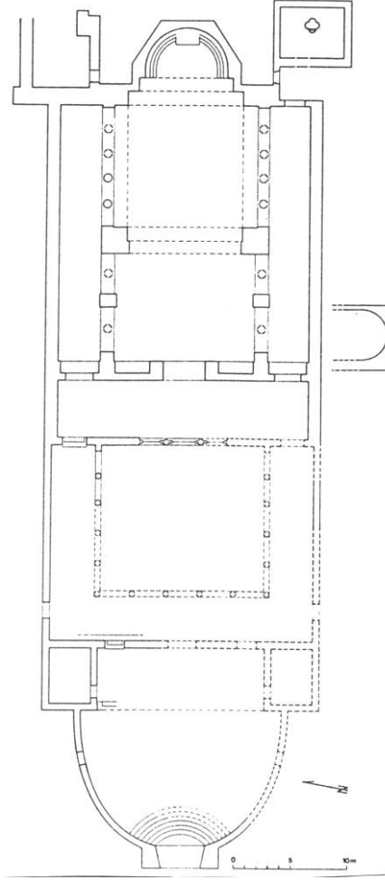
Çiz. 3- Meryemlik, Kubbeli Kilise planı (F. Hild- H. Hellenkemper-G. Hellenkemper-Salies, "Kommagene-Kilikien-Isaurien", RBK IV, 1990, 236, Abb. 21)
