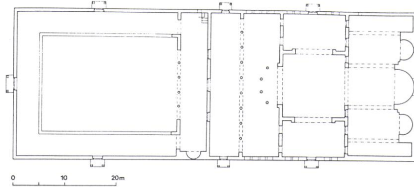
Çiz. 9- Korykos, Mezar kilisesi planı (F. Hild- H. Hellenkemper-G. Hellenkemper-Salies, "Kommagene-Kilikien-Isaurien", RBK IV, 1990, 213-214, Abb. 13)
