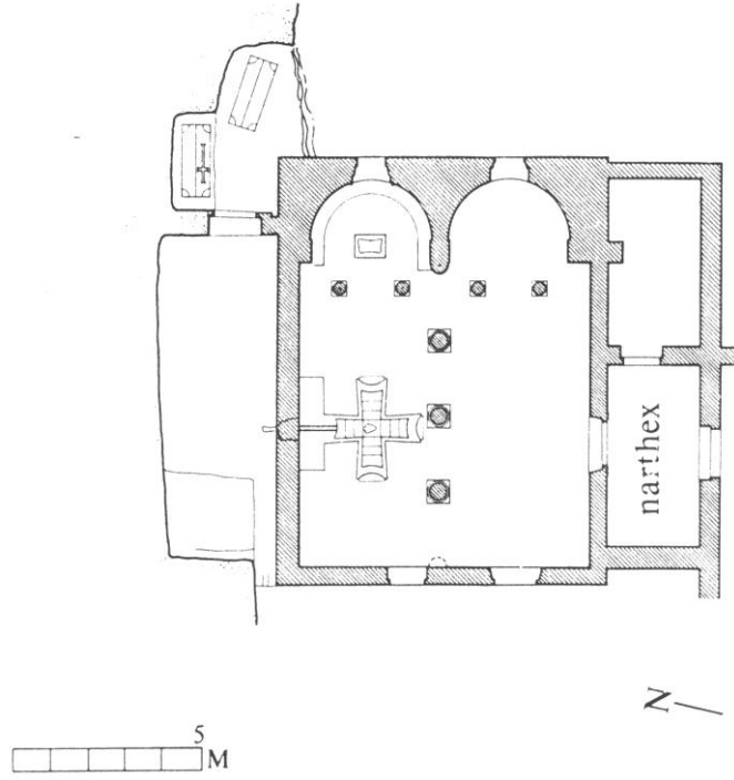
Çiz. 2a-b -Alahan Manastırı vaftiz binasının planı (M. Gough, An Early Christian Monastery in Southern Turkey, 1985, a- Fig. 62; b- Fig. 65.)
