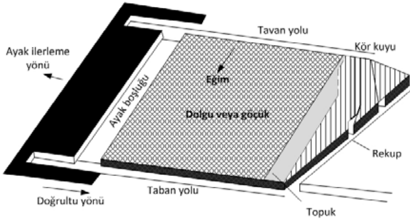
Şekil 1. Uzunayak üretim yöntemi (Şimşir, 2015)
