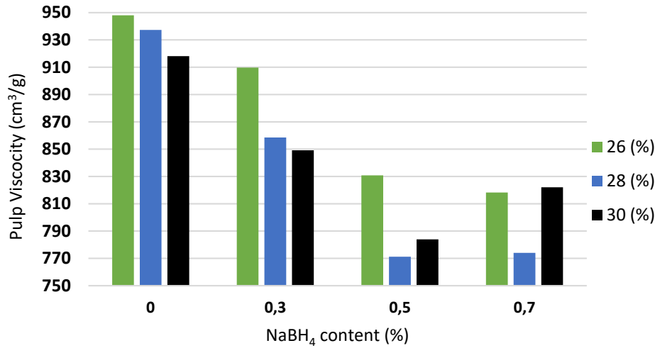
Şekil 1. Montyery çamında Sülfidit ve NaBH 4 ün vizkozite üzerine etkisi Figure 1. The sulfidity and NaBH 4 addition effects on viscosity properties for Monterey pine
