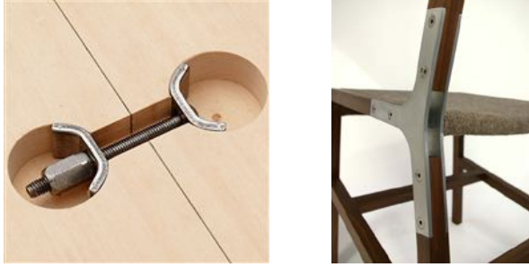
Resim 4.12. Tutkalsız-vida konstrüksiyonlu düz ahşap tabla ve sandalye detayı (26)
