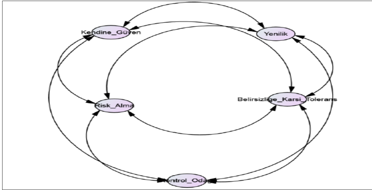
Şekil 2: DFA Modeli
