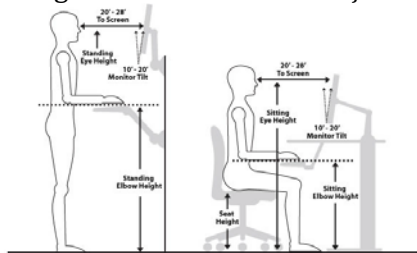
Resim 4.5. Ayakta ve oturarak çalışan bilgisayar kullanıcısı için gerekli bazı ergonomik ölçüler (15)
