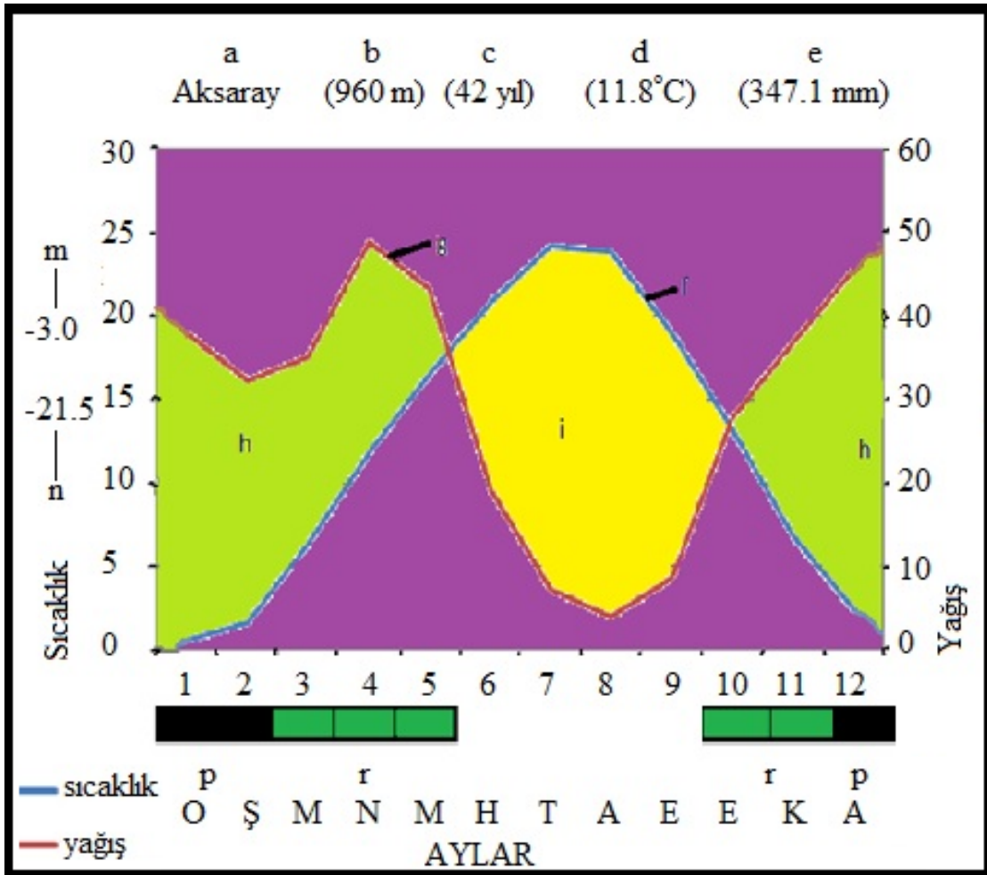
Şekil 2. Aksaray iline ait ombrotermik iklim diyagramı a-istasyon adı, b-istasyon rakımı, c-asat süresi, d-yıllık ortalama sıcaklık, e-toplam yıllık yağış ortalaması, f-yağış eğrisi, g-sıcaklık eğrisi, h-yağışlı dönem, i-kurak dönem, m-en soğuk ayın en düşük sıcaklık ortalaması (°C), n-mutlak minimum sıcaklık (°C), p-mutlak donlu aylar, r-don ihtimali olan aylar.
