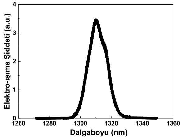
Şekil 3. Dalgaboyuna bağlı elektro-ışınma spektrumu
