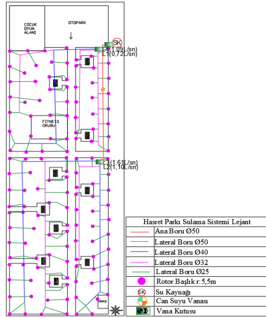
Şekil 3. Hasret Parkı Sulama Sistemi Projelendirmesi
