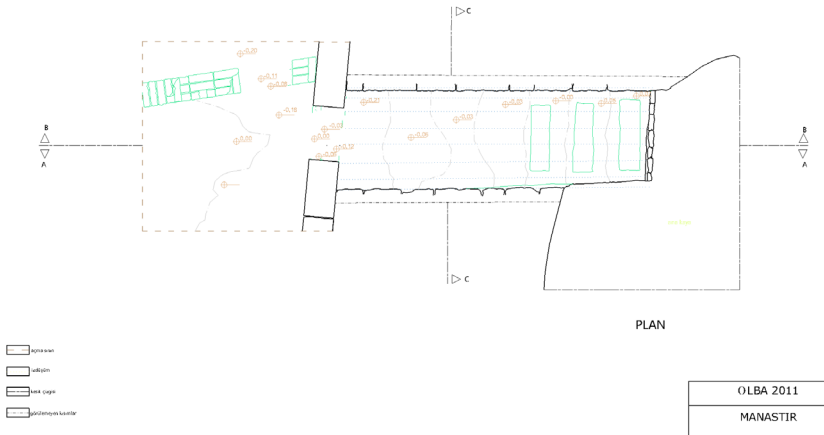
Lev. 9. Olba 2011 Manastır Kazısı (Burak YAZICI - plan, kesit, görünüş) - Model.
