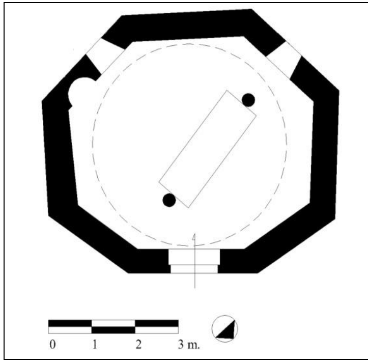
Çizim 1. Hacı Ali Türbesi. Plan (E. Gürsoy 3 ).
