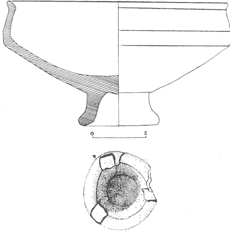
Res. 5 Ortaçağ'a ait sırlı ayaklı tabağın kesiti (üstte) ve dip kısmındaki çömlek fırın desteklerinin görünüşü (altta).
