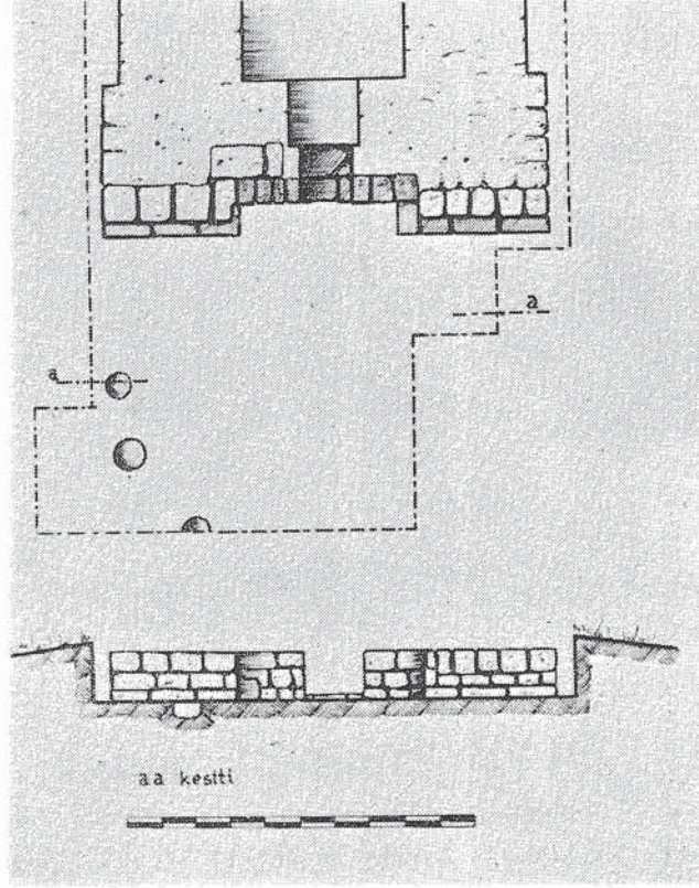
Res. 11 Yukarı kale tapınak cella'sı cephe durum planı ve kuzey-güney kesiti.
