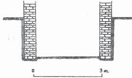
Res. 21 Kaya odasının kuzey-güney kesiti.
