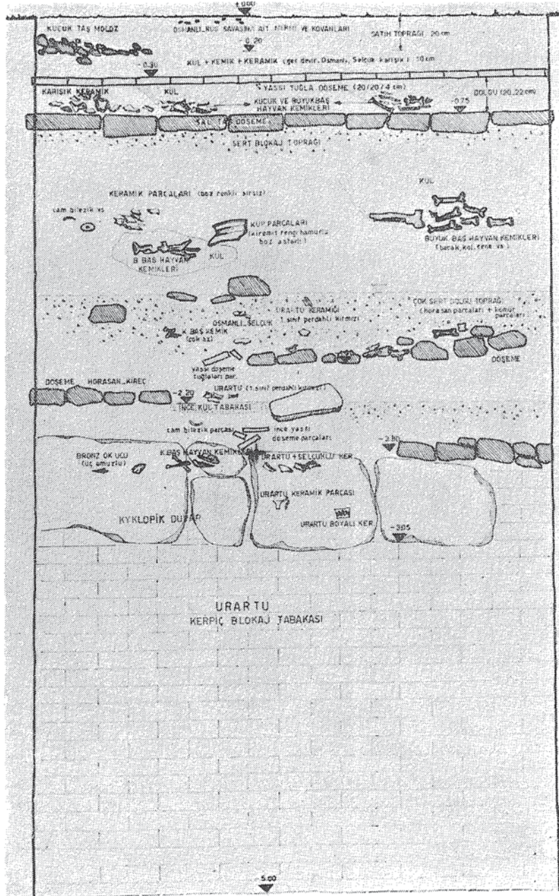
Res. 14 Van kalesi sitadeli açmalarından kesit.
