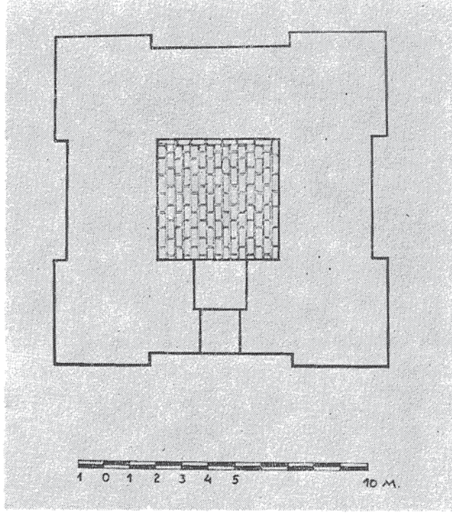
Res. 10 Yukarı kale tapınak cella'sı Urartu çağı temel planı.
