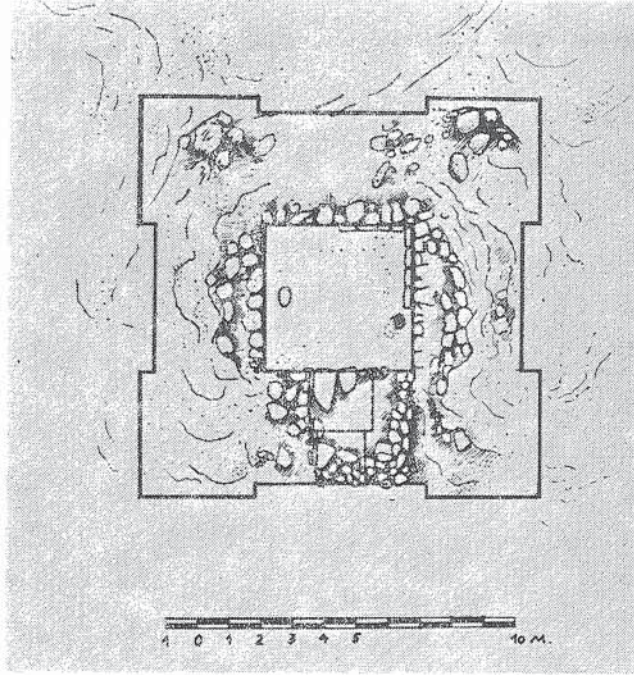
Res. 9 Yukarı kale tapınak cella'sı ve Ortaçağ tadilatı.
