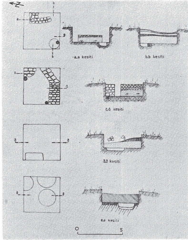
Res. 4 Yukarı kale açmalarının pîan ve kesitleri.
