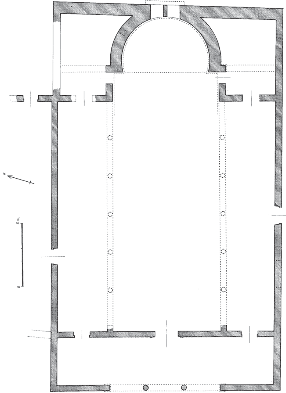
Res. 11 — I. No.lu basilikânın yeni plânı (çizen: Yılmaz Önge).
