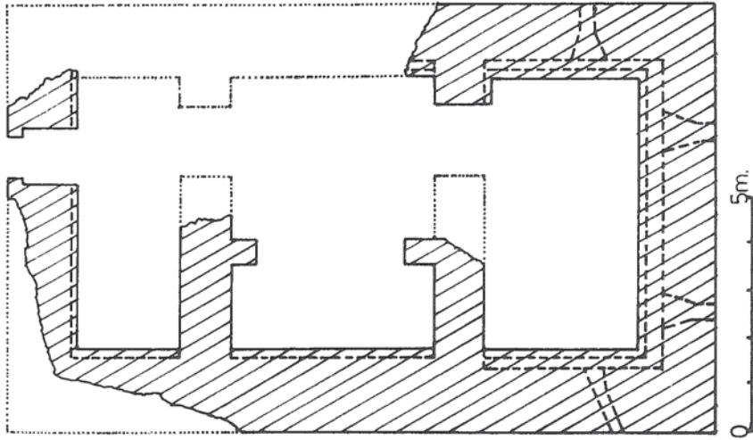
Res. 6 — Hellenistik kulemin plânı (Verzone'den).
