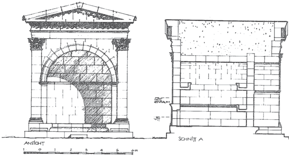
Res. 2 — Aşa'nın mezar anıtının rölövesi (Machatschek'den).
