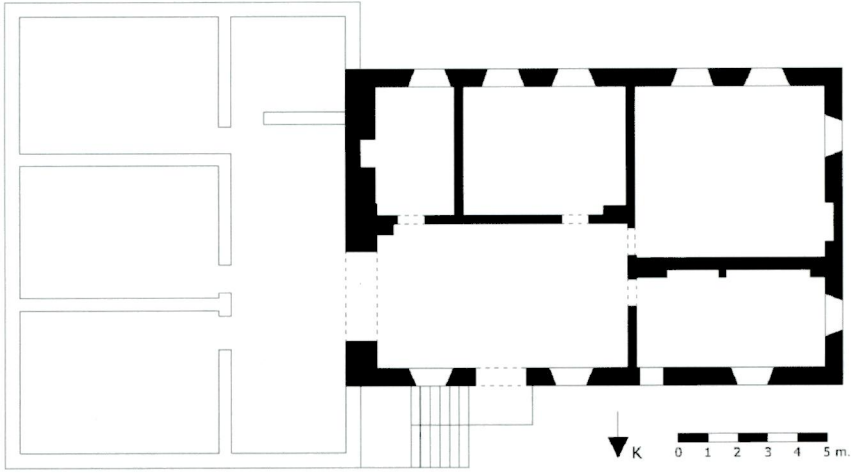
Çizim 1 - Kayseri Safa Mektebi rölöve plâni.
