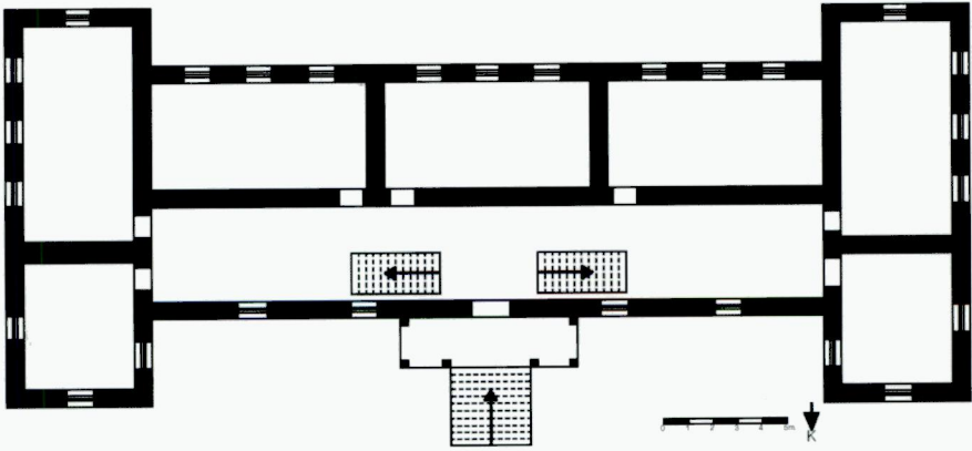
Çizim 11 - Pazarören Köy Enstitüsü (Öğretmen Okulu) planı.
