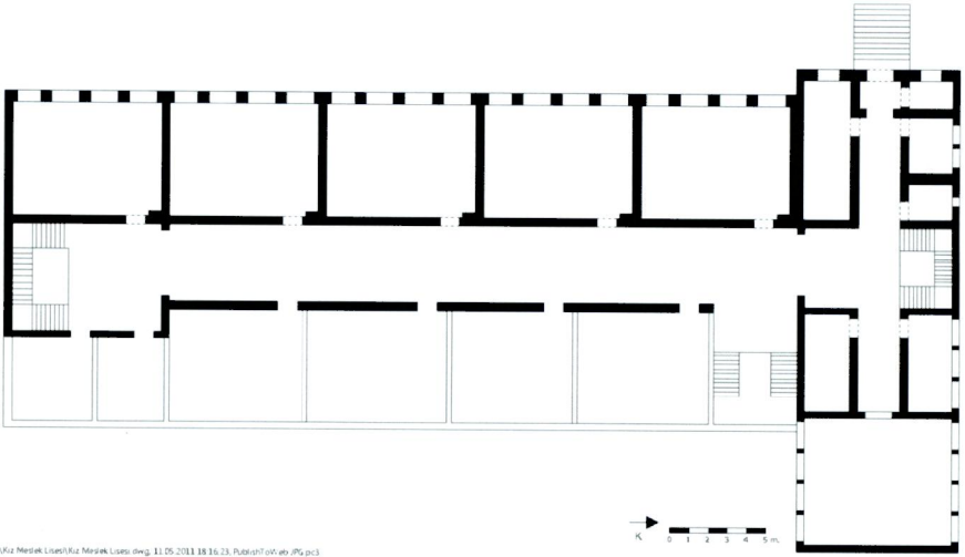
Çizim 12 - Kayseri Kız Meslek Lisesi plânı.
