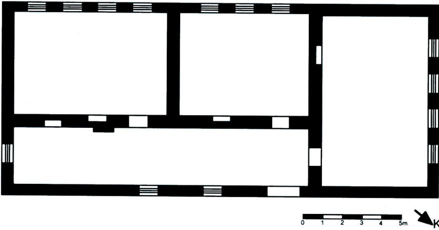
Çizim 17 - Turan (Dimitre) Köyü İlkokulu plânı.
