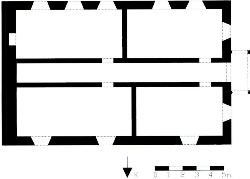
Çizim 1a - Kayseri Safa Mektebi restitüsyon plâni.
