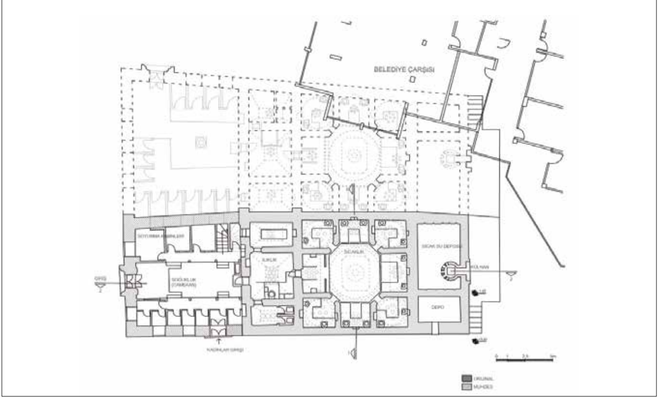
Şekil 19. Hamamın çifte hamam olması durumunda muhtemel yapı / The possible structure of the twin hammam (Restitüsyon Projesi, Kücükaya, 1989).
