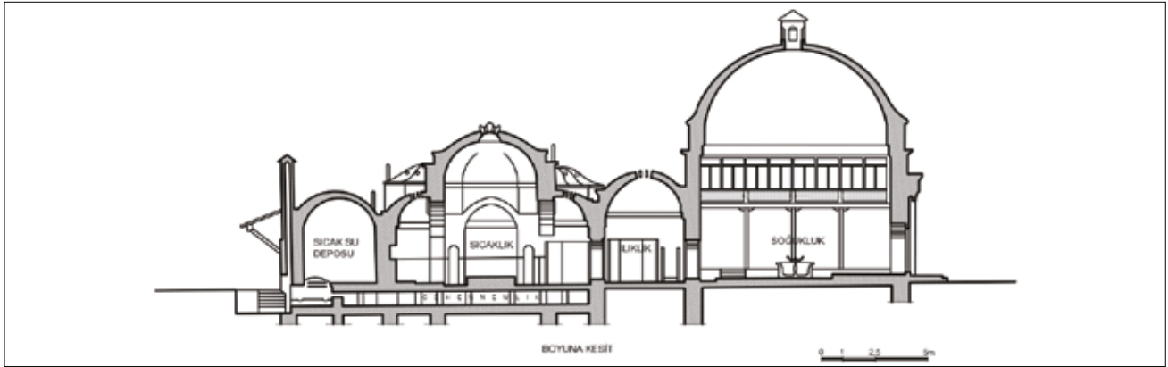
Şekil 18. Sıcaklık, ılıklik ve soğukluk kısımlarının muhtemel boyuna kesiti-restitüsyonu projesi / Longitudinal section of the restitution project showing the hot, warm and cold parts (Küçükçaya, 1989).
