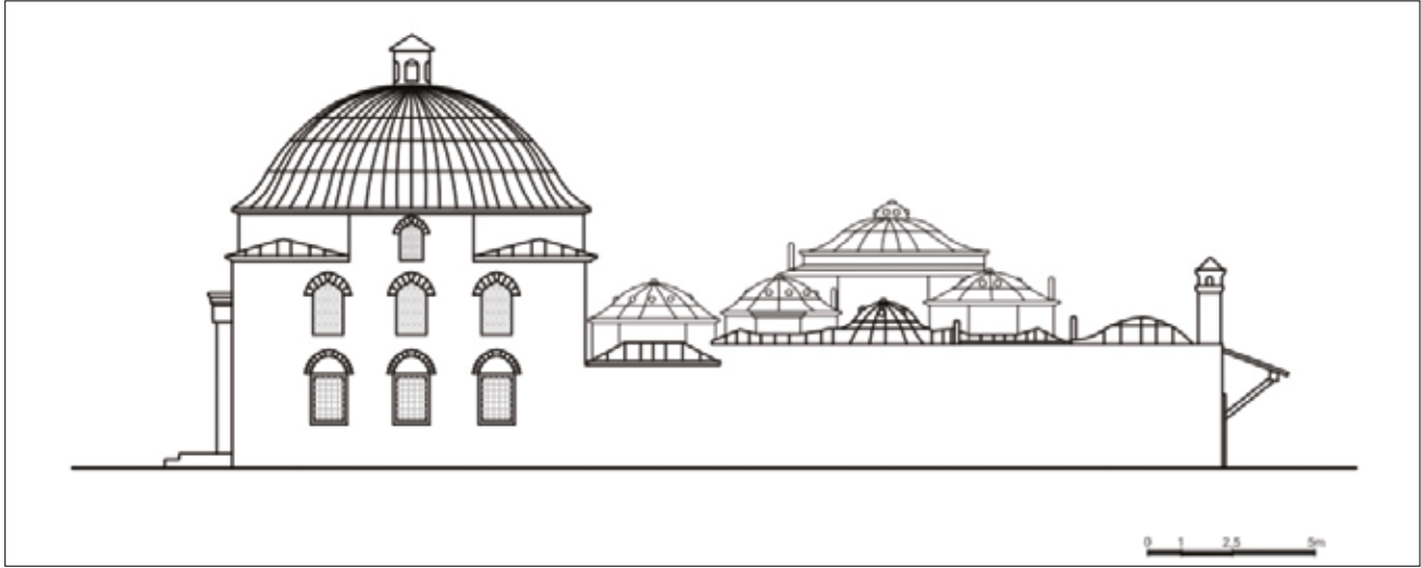
Şekil 15. Hamam doğu cephesi restitüsyon projesi / The Hamam's east facade - restitution project (Küçükaya, 1989).
