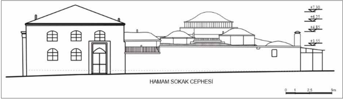
Şekil 14. Hamam doğu cephesi 1989 restorasyonu öncesi durumu / The east facade of the hamam, the restoration of 1989. (TÜMFRA, 1989).
