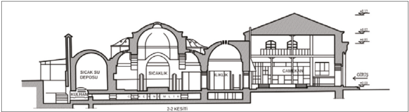
Şekil 17. Çehennemlik, külhan, sıcaklık, ılıklik ve soğukluk kısımlarını gösteren kesit rölövesi / The measured drawing of the section showing the underground hot air channels called çehennemlik, the furnace called külhan, the hot part called sıcaklık, the warm part called ılıklik and the cold part called soğukluk. (TÜMFRA, 1989).
