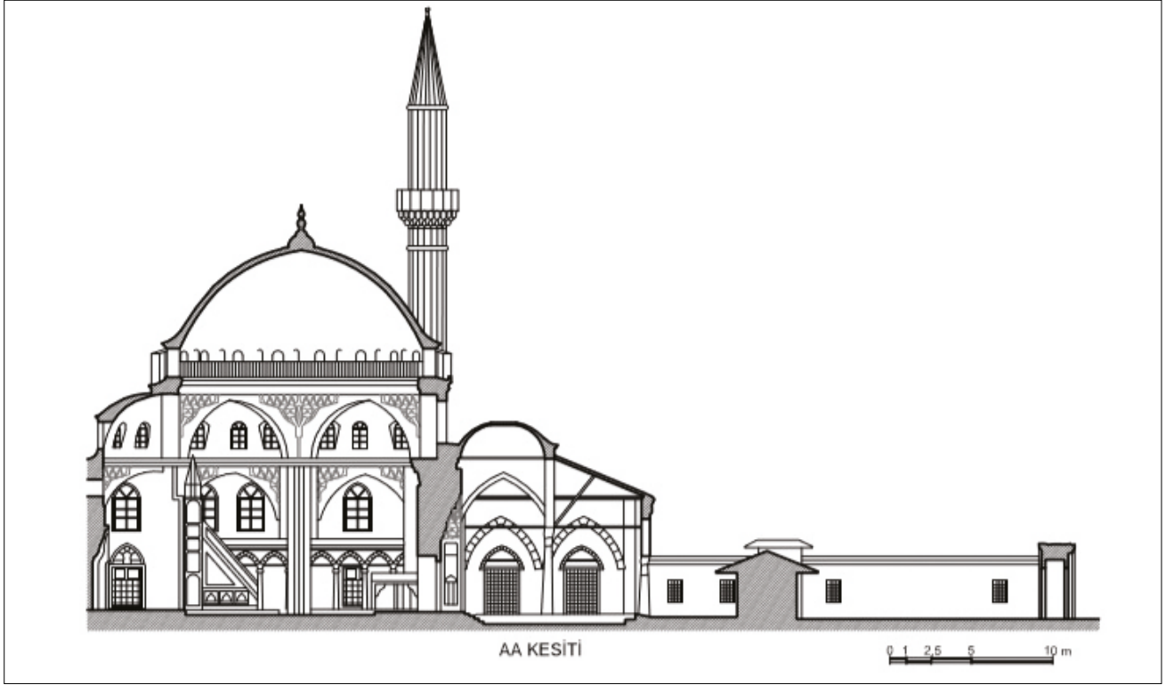
Şekil 9. Babaeski Semiz Ali Paşa Cami ve Avlusu boyuna kesit- rölöve / Longitudinal section of the Babaeski Semiz Ali Paşa Mosque and Courtyard –architectural survey (TÜMFRA, 1989).
