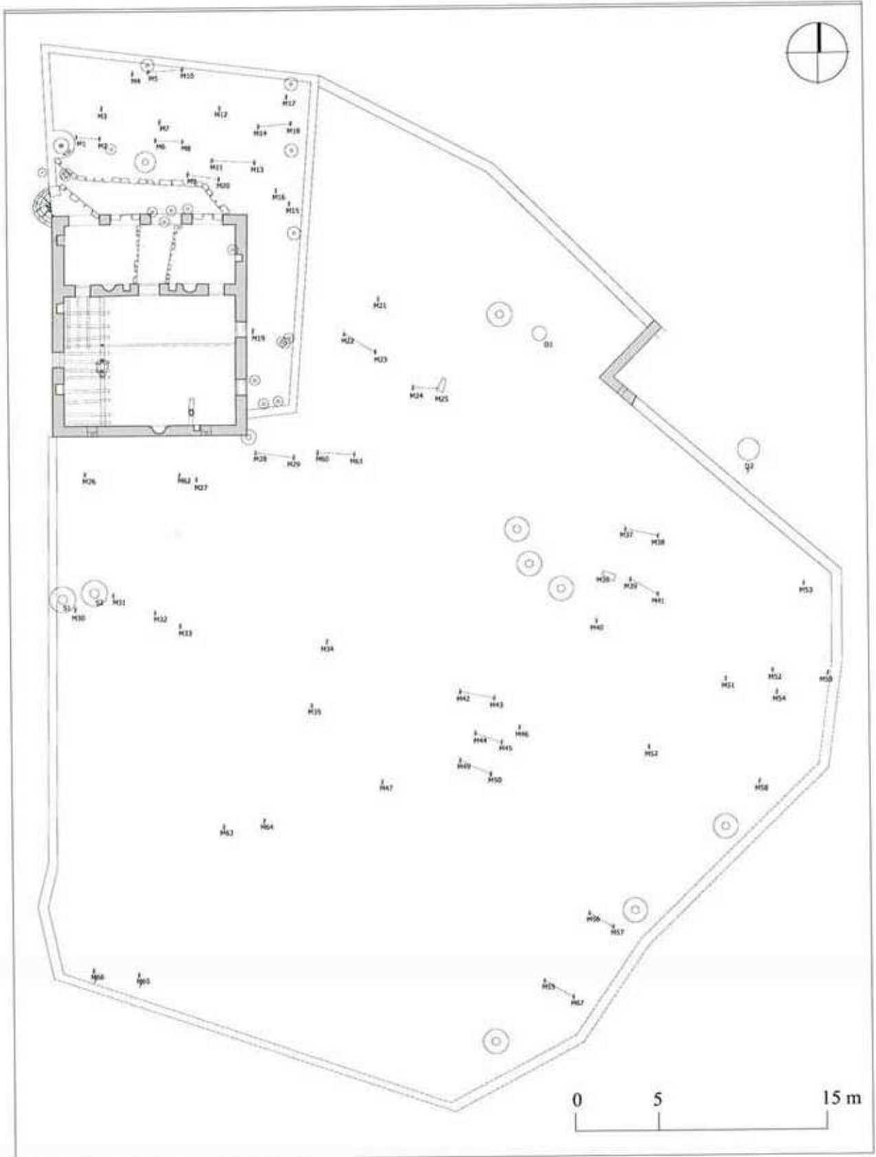
Şek. 1. Çullu köyü: Cami (env. no. K16.C5.1), Hazire ve Doğu Mezarlığı, rölöve planı.
