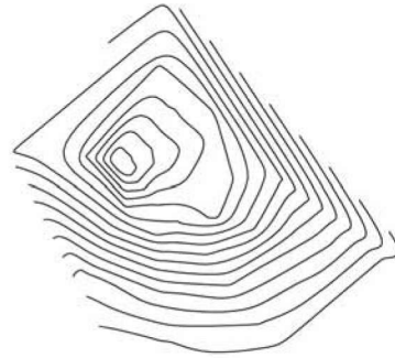
Şek. 3. Taşlı Höyük 2 güney cepheden görünüş. (env. no: N36.A9.89).
