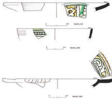
Şek. 1. Taşlı Höyük 1'de (env. no: N36.A9.44) bulunan kap parçaları.
