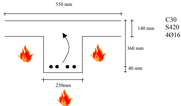
Şekil 8. Tablalı kesite ait kesit ve malzeme özellikleri
