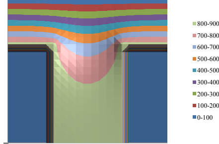
Şekil 9: Tablalı kesitte sıcaklık dağılımı
