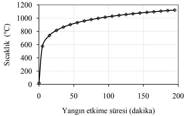
Şekil 7. ISO834 sıcaklık yangın etkime süresi
