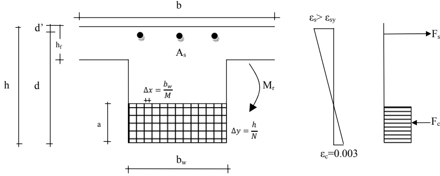
Şekil 6. Basınç bölgesinin tablalı kesitin alt bölgesinde olması durumunda (mesnette) tablalı kesitte oluşan kuvvetler
