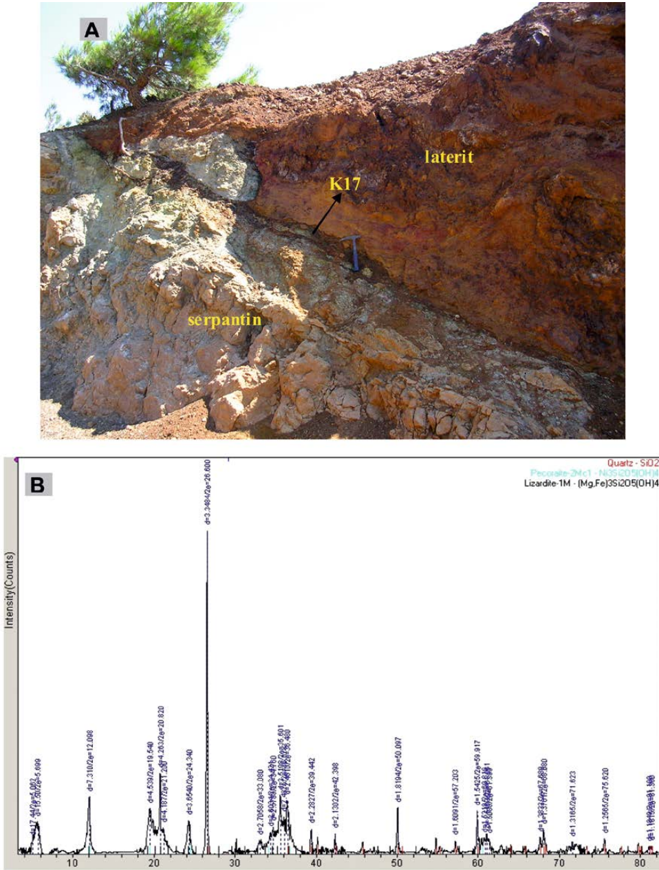
Şekil 14. Çaldağ Ni-Co yatağı Kuzey Ocağı'nda, serpantinleşmiş ultrabazik ile lateritin sınırını oluşturan fay zonunda gelişen pecoraite (K-17) oluşumlarının arazi fotoğrafı (A) ve XRD analizi (B).
