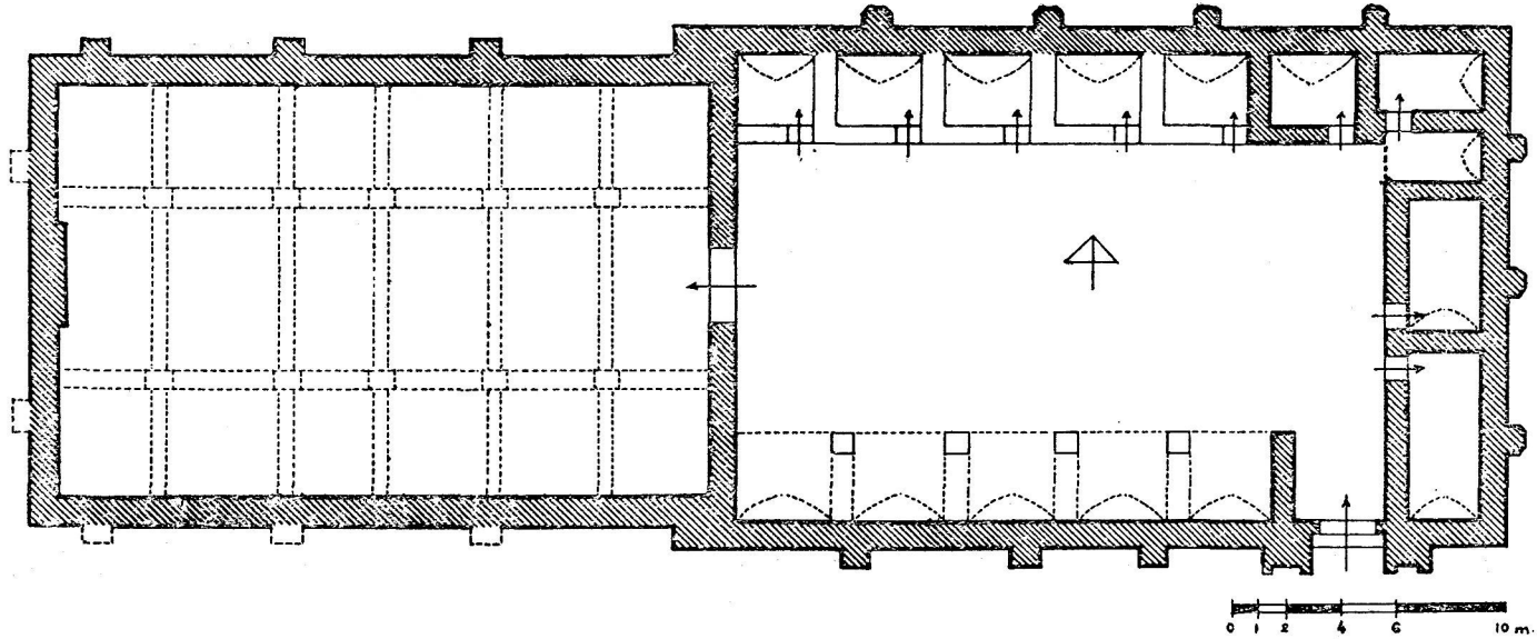
Şek. 5 - Çingene Hanı'nın, Sayın Celâl Yalvaç'ın aldığı ölçülere göre çizilmiş planı.
