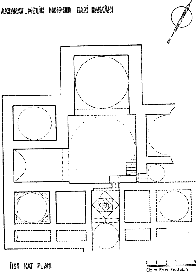
Şek. 2- Aksaray - Melik Mahmud Gazi Hangâhı, birinci kat planı. (Rölöve ve çizim R. Eser Gültekin 1992.)
