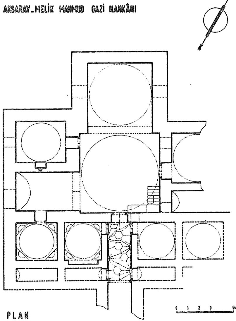
Şek. 1- Aksaray - Melik Mahmud Gazi Hangâhı, Zemin kat planı. (Rölöve ve çizim R. Eser Gültekin 1992.)
