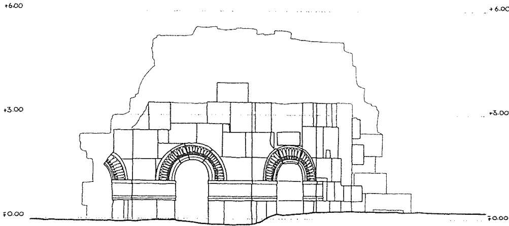
DOĞU CEPHE 1/50 EKİM 96
