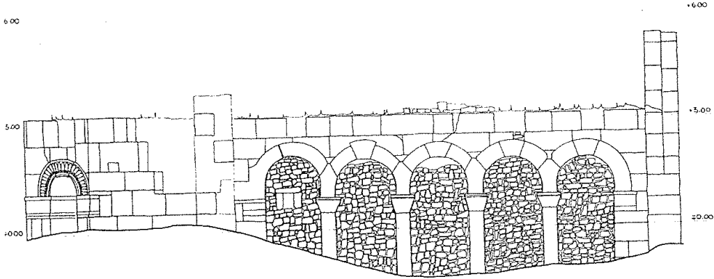
KUZUY NEF GÜNEYE BAKIŞ 1/50 EKİM 96
