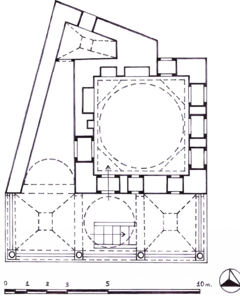
Şek.2- Ahmediye Kütüphanesi Planı (A.Şahin'den işlenerek).
