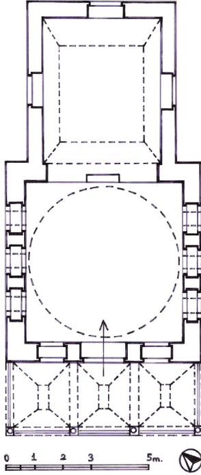
Şek.4- Hacı Selim Ağa Kütüphanesi Planı (B.Ünsal'dan işlenerek).
