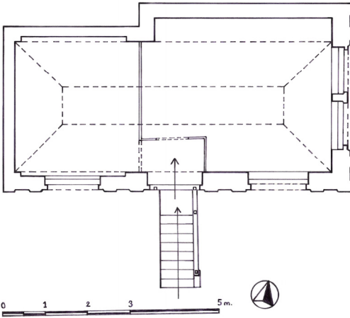
Şek.6- Aziz Mahmut Hüdayi Külliyesi (Lütfi Bey) Kütüphanesi Planı (H.S. Ünal).
