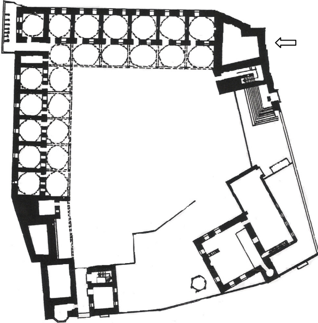
Şek.1- Ahmediye Külliyesi Planı (VGM.'nden).
