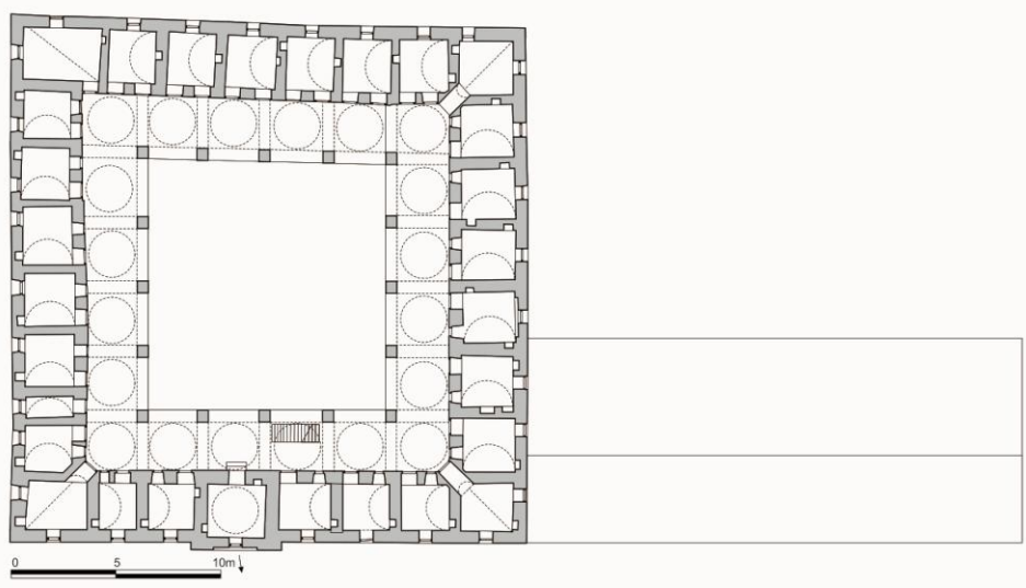
Plan 2- Çukur han, üst kat restitüsyon planı.
