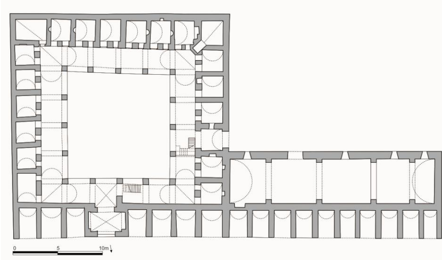
Plan.1- Çukur Han, zemin kat restitüsyon planı
