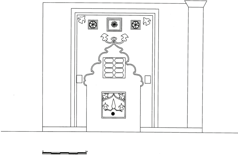
Şek.2- Bozcaada Namazgah Meydanı Çeşmesi doğu cephe elevasyonu
