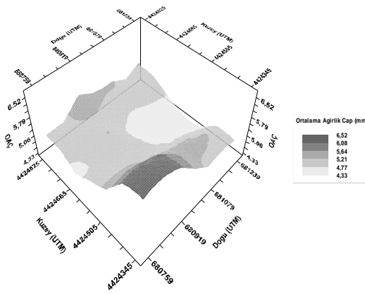
Şekil 11- Ortalama ağırlık çap değerlerine ait dağılım haritası. Figure 11- Spatial distribution patterns of mean weight diameter
