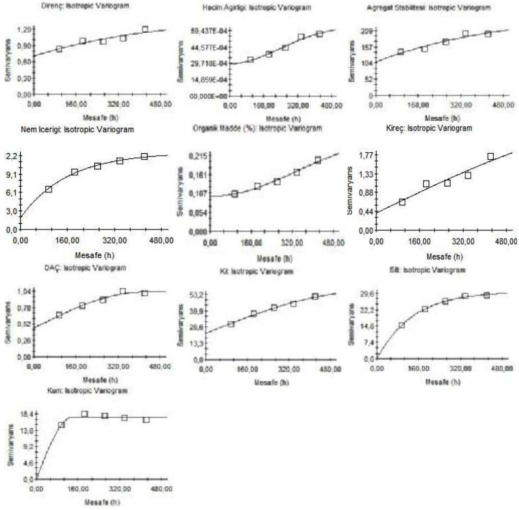
Şekil 4- Deneysel semivaryanslar ve semivariogram modelleri
