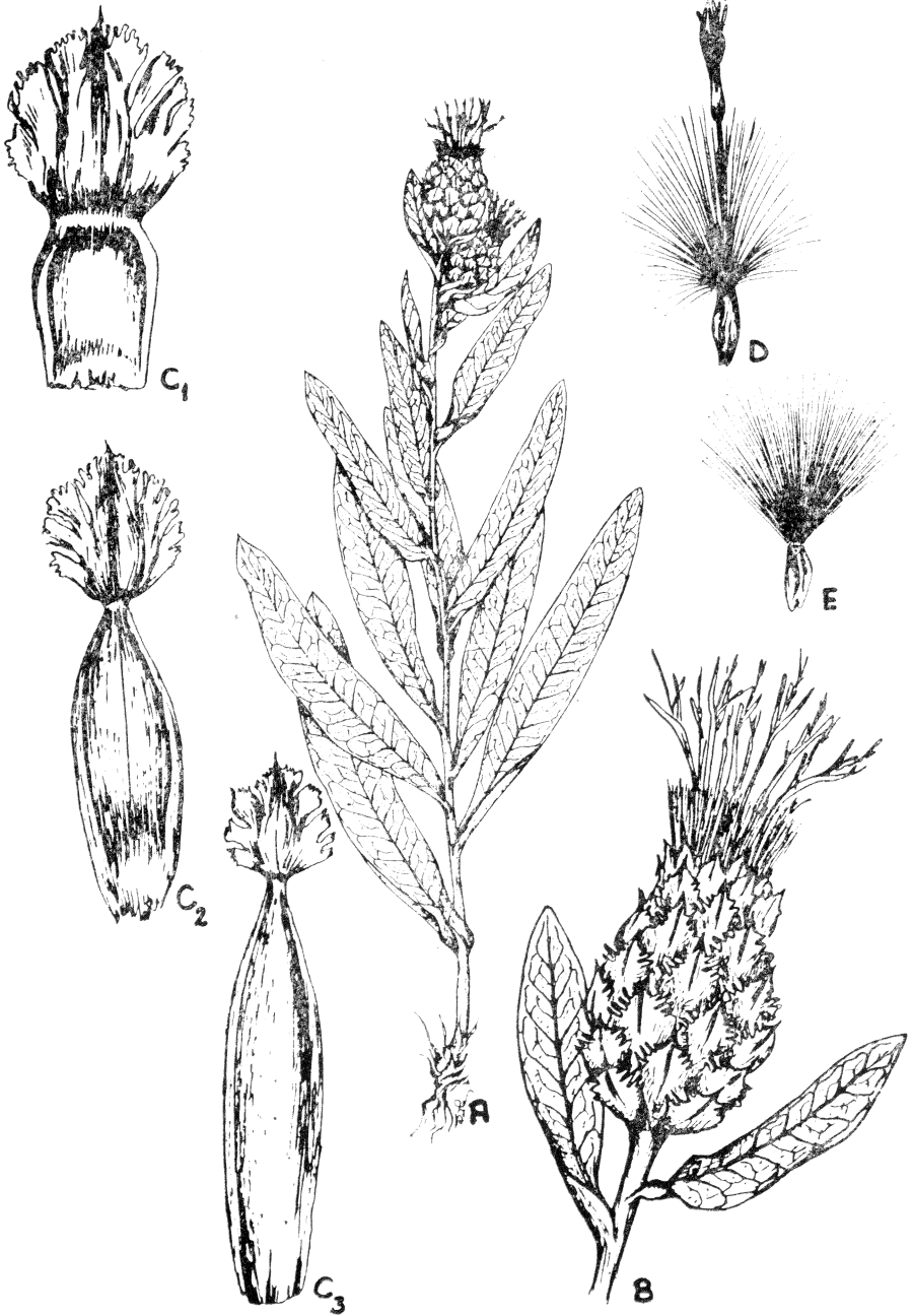
Şekil 2: Centaurea saligna (C. Koch) Wagenitz. A. Genel görünüş; B. Kapitulum ( \times 2 ); C. İnvokrum brakteleri ( \times 3 ); C 1 (Alt), C 2 (Orta), C 3 (Üst); D. Tek bir çiçek ( \times 2 ); E. Aken ( \times 2 ).
