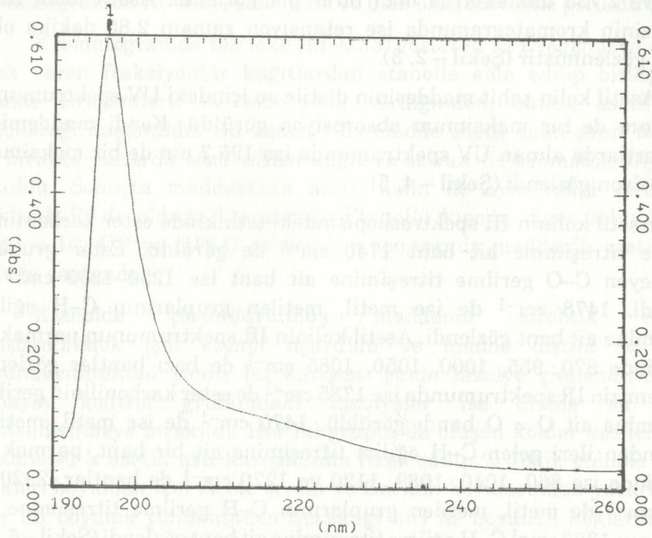
Şekil - 4 : Asetil kolinin UV spektrumu.
