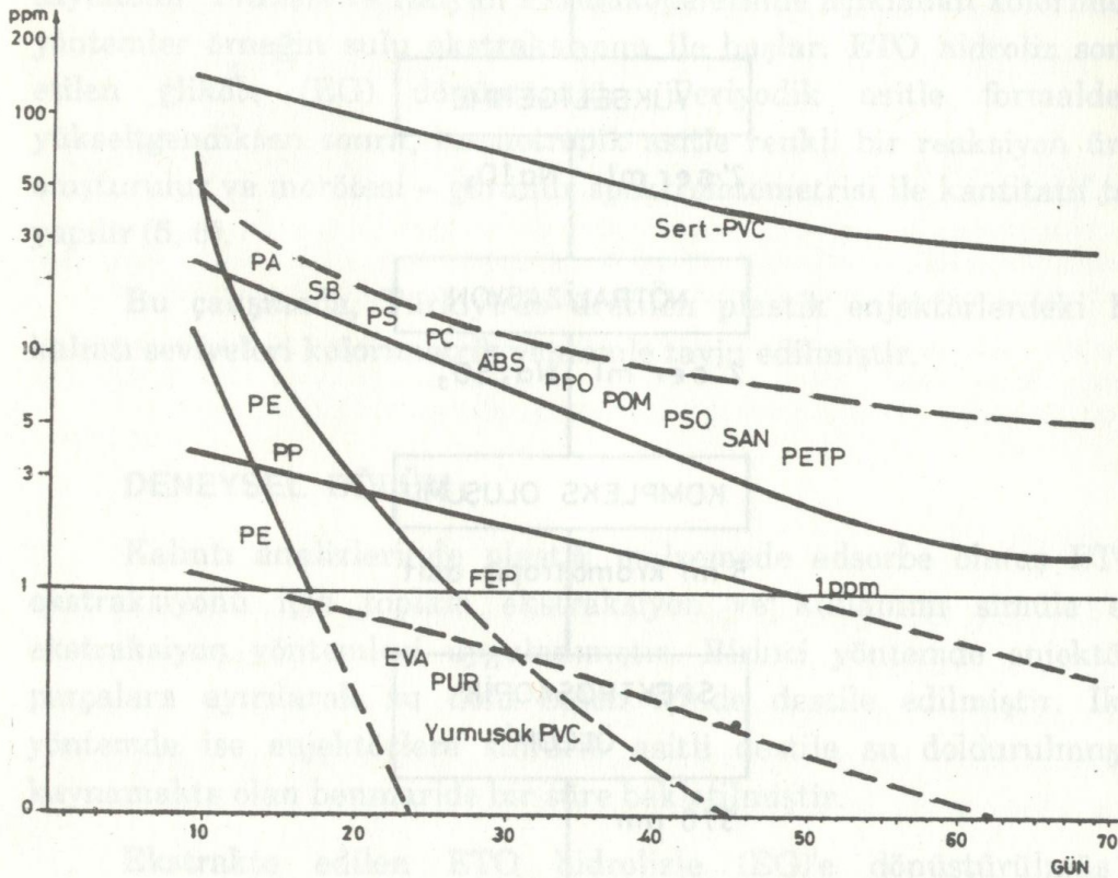
Şekil - 2 : Plastik Malzemelerin ETO Dezorpsiyonu.
