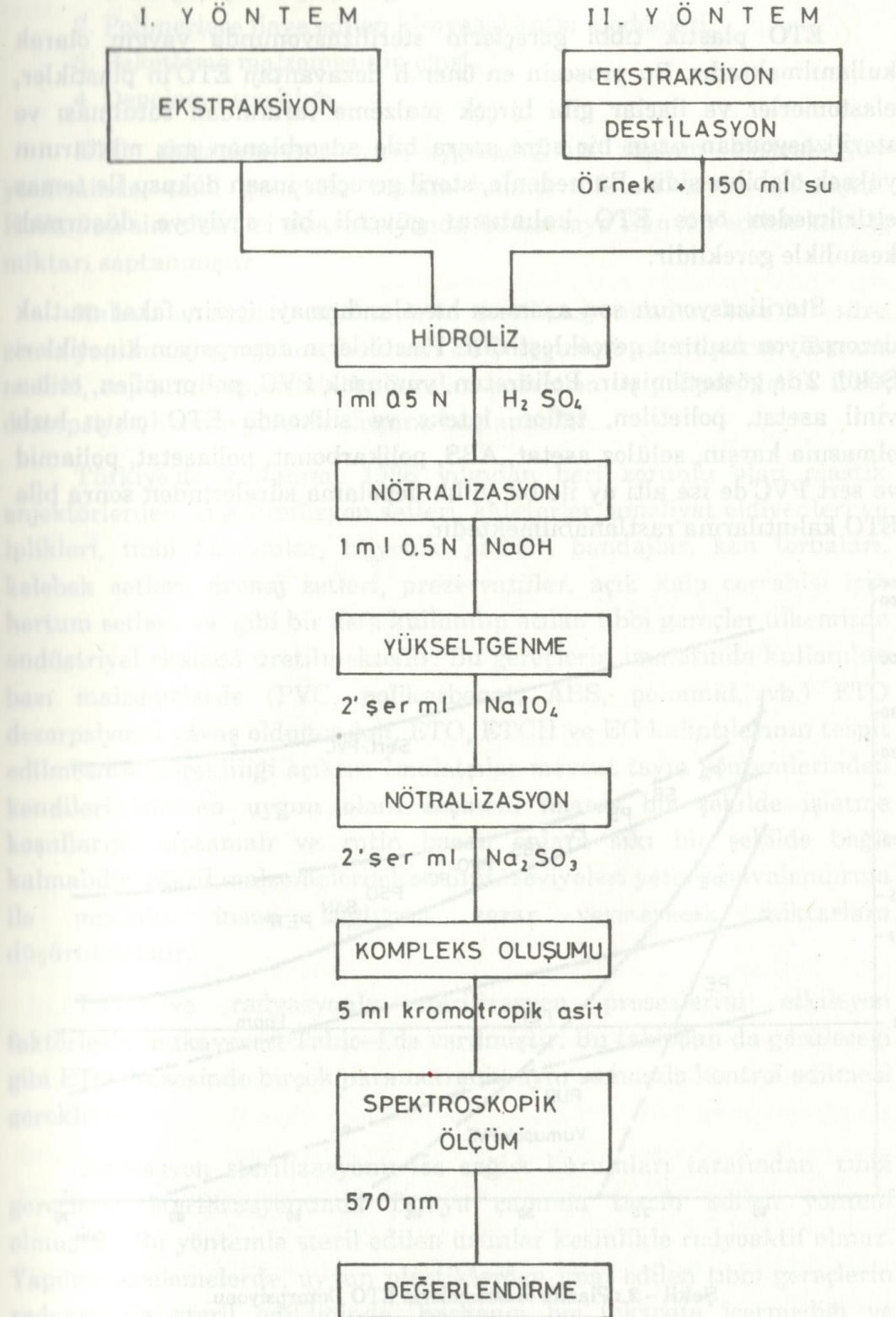
Şekil - 1 : ETO analizi akış diyagramı.
