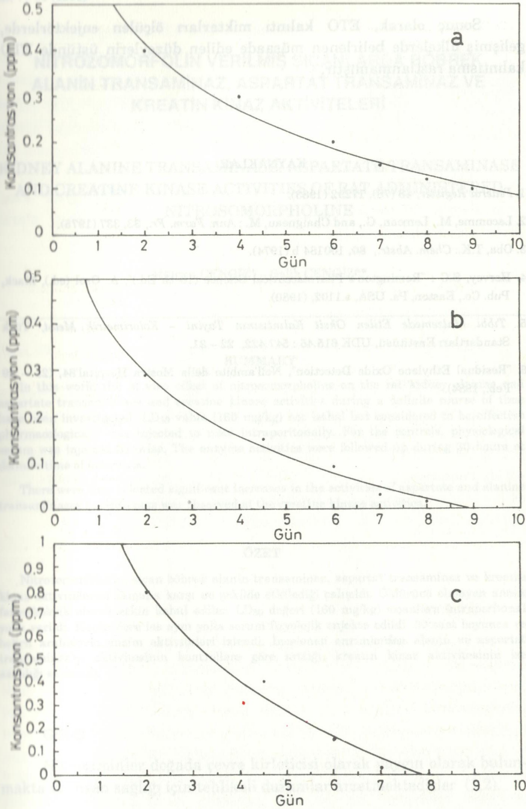
Şekil - 3 : Enjektörlerdeki etilen oksit miktarlarının zamanla değişimi. II. Yöntem:
