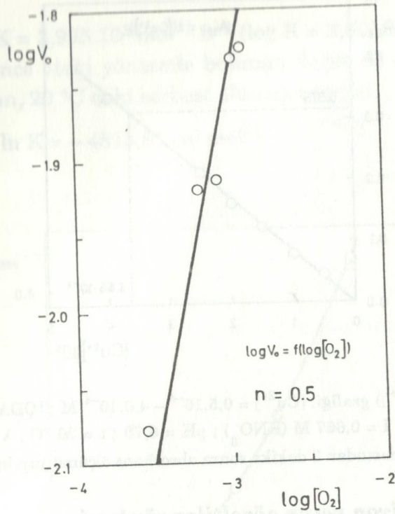
Şekil - 6 : Reaksiyon hızı üzerine oksijen konsantrasyonunun etkisi. [ODAK] = [Cu 2+ ] = 8,0 · 10 -4 M ; I = 0,40 M (KNO 3 ) ; pH = 6,52 ; t = 25 °C ; λ = 560 nm.
