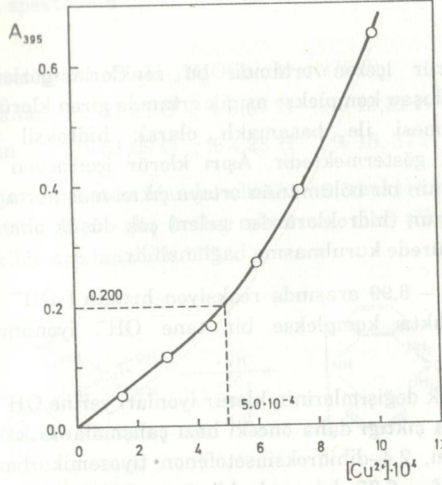
Şekil - 8 : Seyrelme eğrisi. [\text{ODAK}] = [\text{Cu}^{2+}] = 1,5 \cdot 10^{-4} - 10,0 \cdot 10^{-4} \text{ M} ; I = 0,50 \text{ M (KNO}_3) ; \text{pH} = 6,70 ; t = 20^\circ \text{C} ; \lambda = 395 \text{ nm} ; metal iyonunun katılmasından 3 dakika sonra absorbans ölçümü yapılmıştır.
