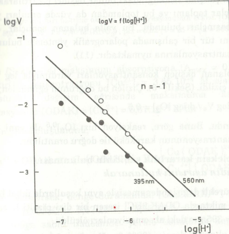
Şekil - 5 : Reaksiyon hızlarının pH'a bağlı olarak değişimi. [\text{ODAK}] = [\text{Cu}^{2+}] = 8,0 \cdot 10^{-4} \text{ M} ; I = 0,40 \text{ M (KNO}_3) ; t = 20 \text{ }^\circ\text{C} ; \lambda = 395 \text{ nm} ve \lambda = 560 \text{ nm} .
