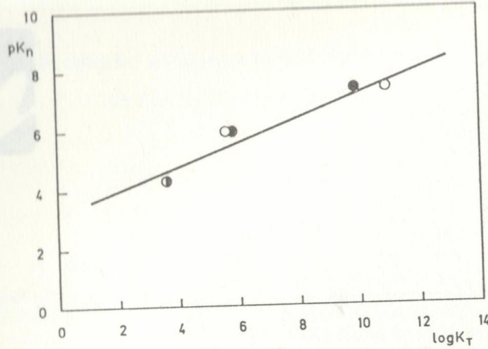
Şekil - 10 : pK_n = f(\log K_T) grafiği. Eşit absorpsiyon yöntemiyle bulunan kararlılık sabitleri siyah noktalarla gösterilmiştir. 2,2'-diaminokarbonilid için \log K_T = 3,602 ve 3,601 ; 3,3'-diaminokarbonilid için \log K_T = 5,615 ve 5,833 (17) ; 4,4'-diaminokarbonilid için \log K_T = 10,954 ve 9,999 (18).
