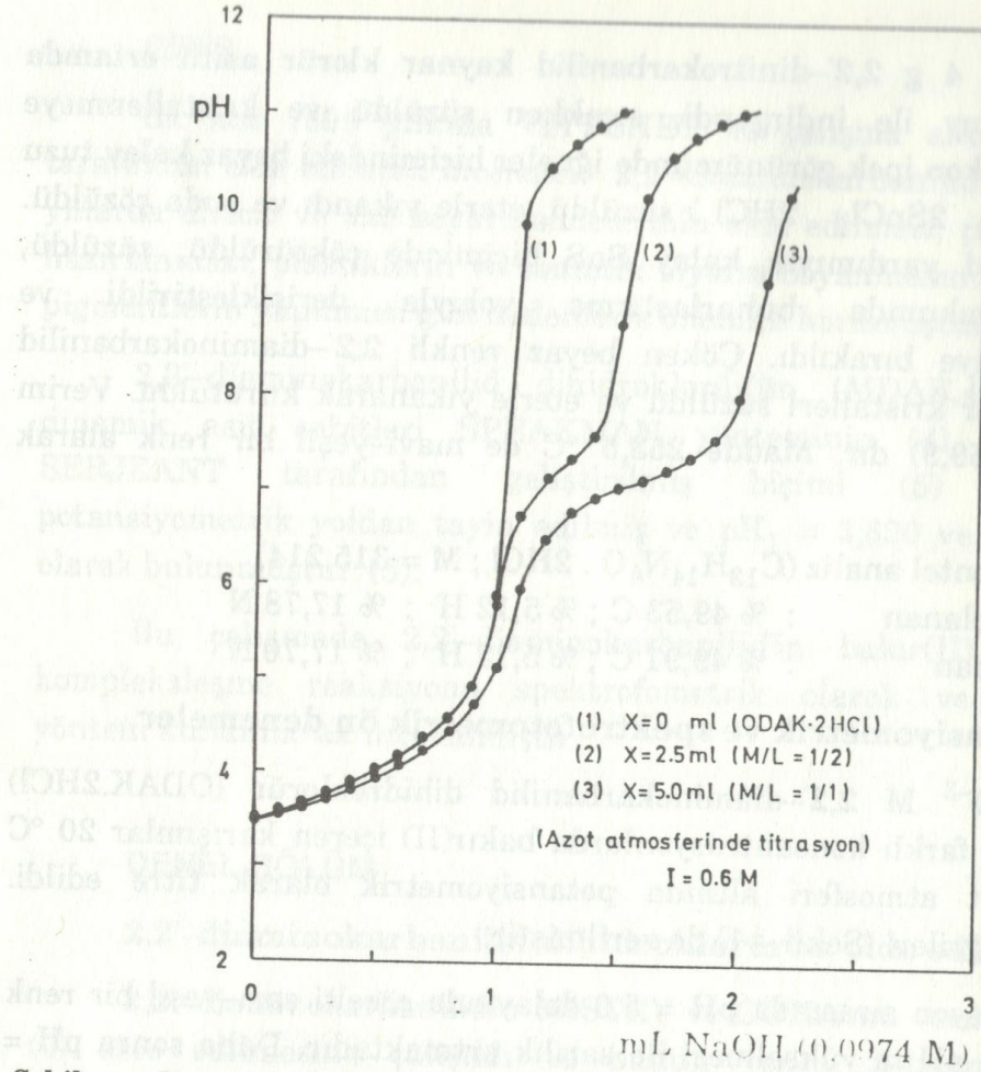
Şekil - 1 : Potansiyometrik titrasyon eğrileri. [ODAK] = 1,0 \cdot 10^{-3} M ; [Cu^{2+}] = 5,0 \cdot 10^{-4} M (X = 2,5 mL) ; [Cu^{2+}] = 1,0 \cdot 10^{-3} M (X = 5,0 mL) ; I = 0,60 M ( KNO_3 ) ; t = 20°C.
