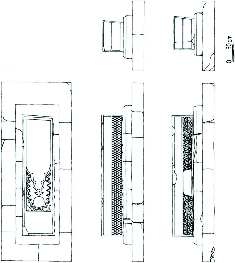
Resim 19 — Göç 33 no'lu mezarın rölövesi.
