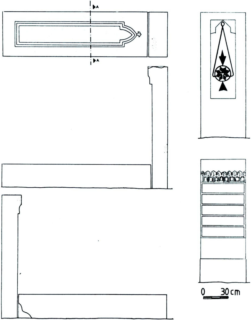
Resim 12 — G029 no'lu mezarın rölövesi.
