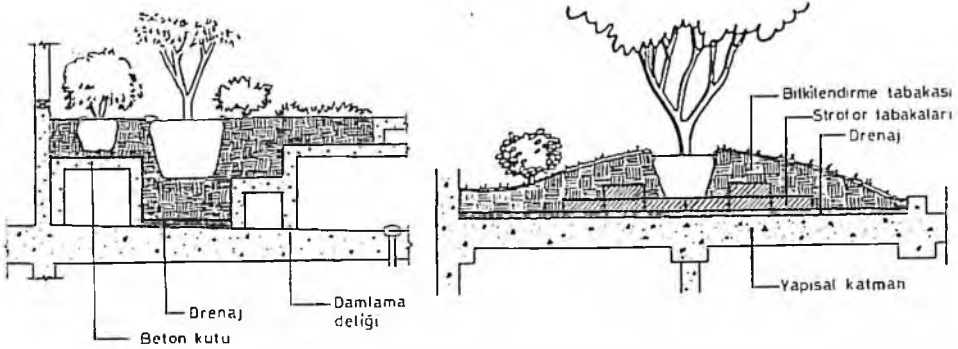
Şekil 9: Beton Kutular ya da Strofor Tabakaları Kullanılarak Ağırlığın Azaltılması
