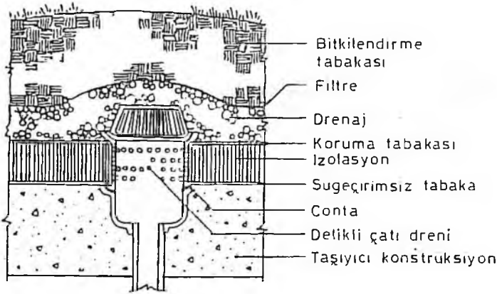
Şekil 2: Bitkilendirme Tabakasının Altında Çatı Dreni
