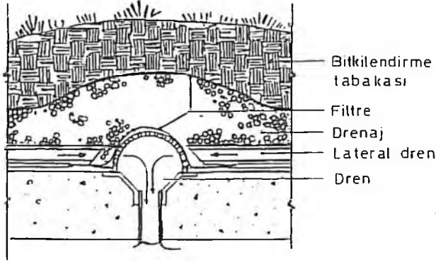
Şekil 6: Bitkilendirme Tabakasının Altında Yer Alan Ana Çatı Dreni
