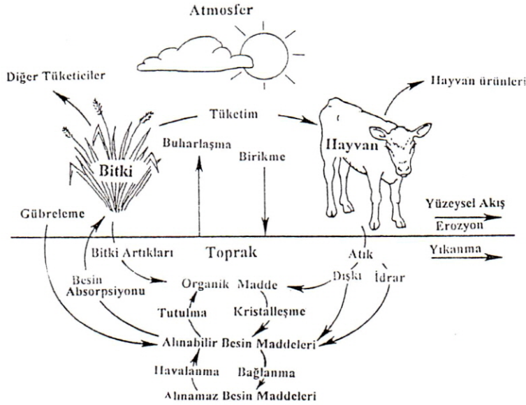
Şekil 1: Otlak ekosistemindeki besin döngüsü (HEITSCHMIDT/STUTH 1991'den alınmıştır)
