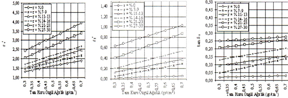
Şekil 10: 9.8 GHz frekanslarında dielektrik sabiti ( \epsilon' ), kayıp faktörü ( \epsilon'' ) ve kayıp tanjantının ( \tan \delta ) miktarının fonksiyonu olarak kayıp tanjantının özgül ağırlıkla değişimi.
