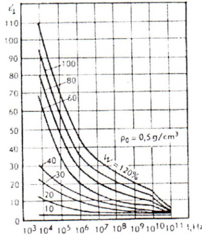
Şekil 3: Rutubetli odunun liflere dik yöndeki dielektrik sabitinin \epsilon'_{\perp} frekansla değişimi ( t = 20^{\circ}\text{C} ), W: rutubet miktarı.
