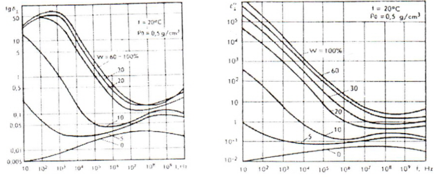
Şekil 4 : Rutubetli odunun liflere dik yöndeki dielektrik kayıp faktörünün \epsilon''_{\perp} ve kayıp tanjantının \tan \delta frekansla değişimi ( t = 20^{\circ}\text{C} ); W = rutubet miktarı.
