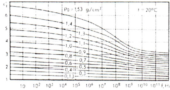
Şekil 1: Hücre çeperi maddesi ve tam kuru odunun liflere dik yöndeki dielektrik sabitinin \epsilon'_{\perp} frekansla değişimi ( t = 20^\circ\text{C} ).
