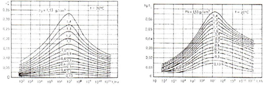
Şekil 2: Hücre çepri maddesi ve tam kuru odunun liflere dik yöndeki kayıp faktörünün \epsilon''_{\perp} ve kayıp tanjantının \tan \delta_{\perp} frekansla değişimi ( t = 20^{\circ}\text{C} ).
