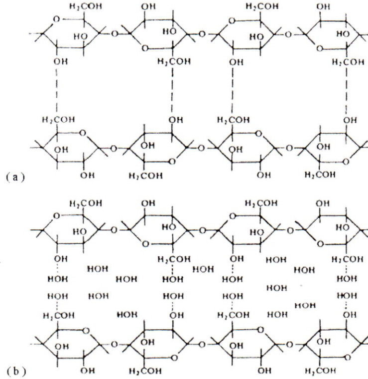
Şekil 9: Selülozün moleküler bağları üzerine rutubetin etkisi; (a) İkincil kuvvetlerle bağlı selüloz makromolekülleri, (b) Su molekülleri tarafından zincirler arası bağların kırılması.
