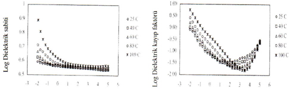
Şekil 5: Düşük frekanslarda liflere paralel yönde tam kuru odunun dielektrik sabiti ve kayıp faktörünün sıcaklıkla değişimi.
