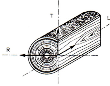
Şekil 8: Odunun 3 ana lif yönü. L, liflere paralel yön; R, radyal yön; T, teğet yön.
