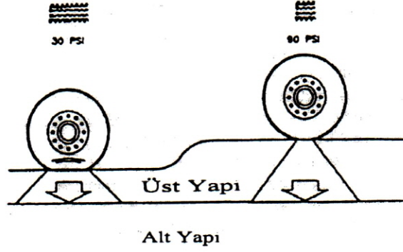
Şekil 6: Lastik hava basıncına göre gerekli altyapı ve üstyapı kalınlıkları ( BROWN/ SESIONS 1995)
