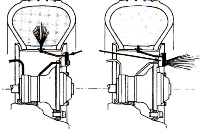
Şekil 2: CTI ile lastiklere hava basılması ve lastiklerden hava boşaltılması.(USDA 1993)
