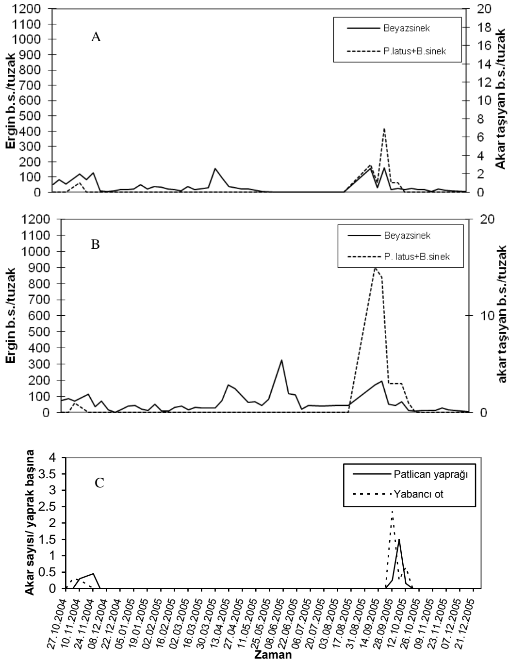
Şekil 2. Patlıcan serası örneklemeleeri A: Patlıcan serası yapışkan tuzak, B: Sera çevresi yapışkan tuzak, C: Yaprak örneklemeleeri.
