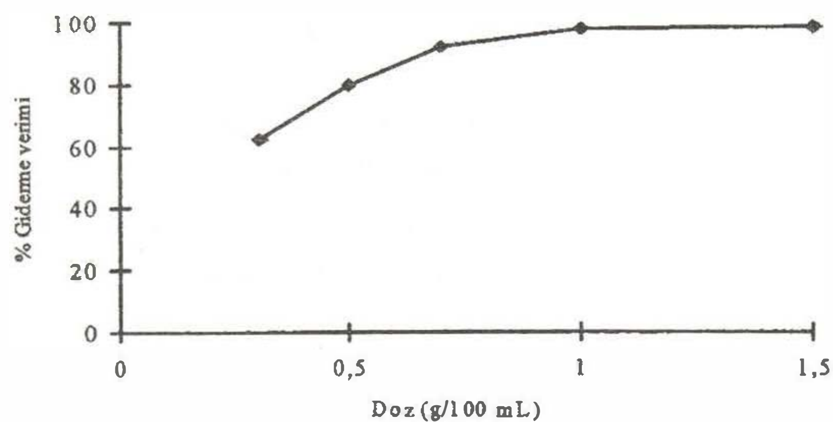
Şekil 3. Cd(II) iyonu adsorpsiyonuna doz etkisi (C 0 : 10 mg/L, t : 60 dak, pH : 6,0, V:100 mL)
