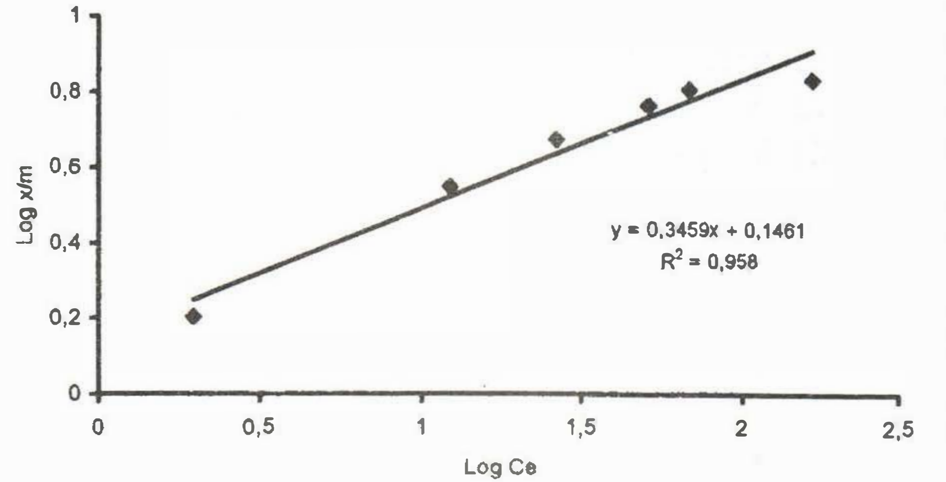
Şekil 7. Freundlich izoterm eşitliği grafiği
