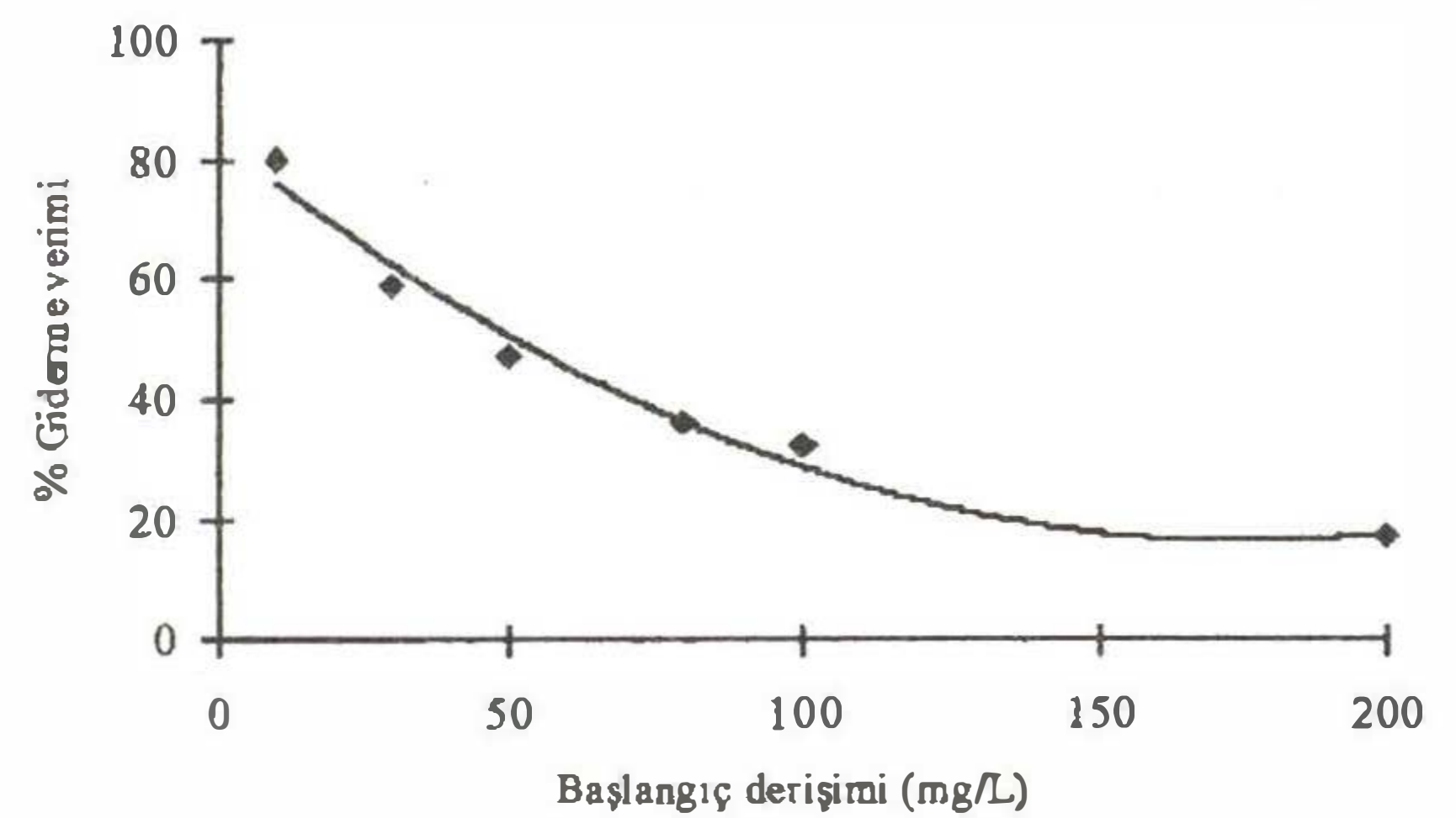
Şekil 5. Cd(II) iyonu adsorpsiyonuna başlangıç derişimi etkisi (Adsorban dozu: 0,5 g/100 mL. çözelti, t : 60 dak., pH : 6,0)
