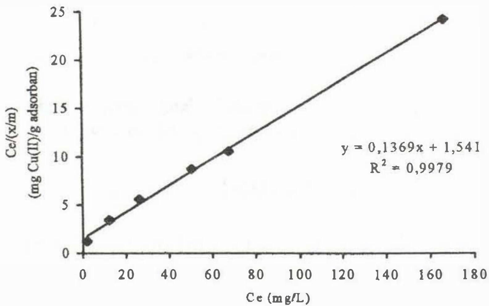
Şekil 7. Langmuir izoterm eşitliği grafiği
