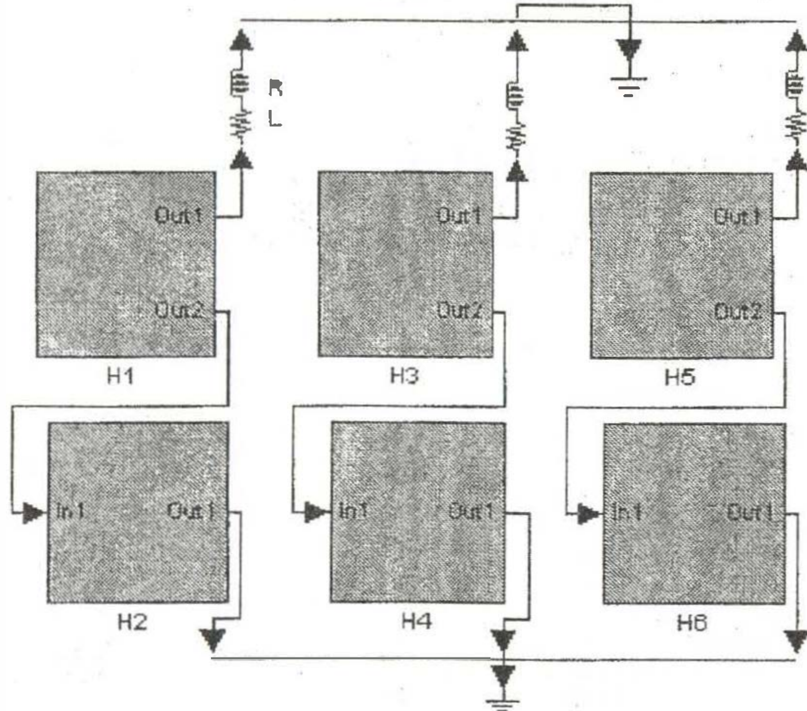
Şekil 8. Üç fazlı, 5-seviyeli kaskat inverter devre modeli
