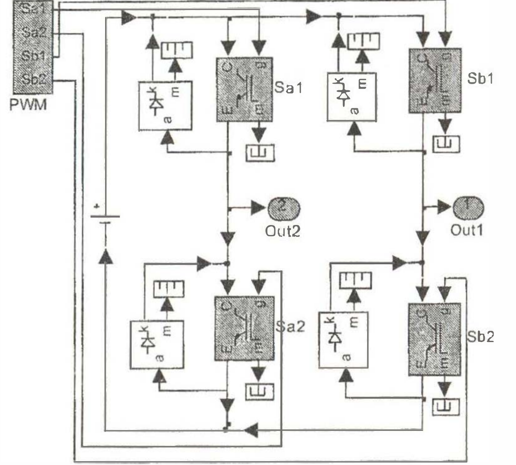
Şekil 9. Tam köprü inverter devre modeli
