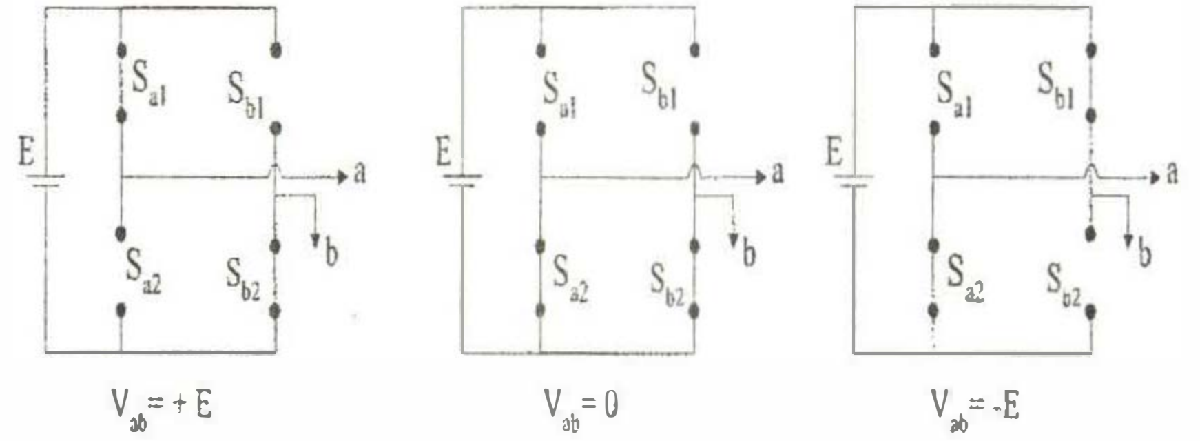
Şekil 1. Bir tam köprü invertere ait anahtarlama durumları ve buna karşılık gelen gerilim seviyeleri.
