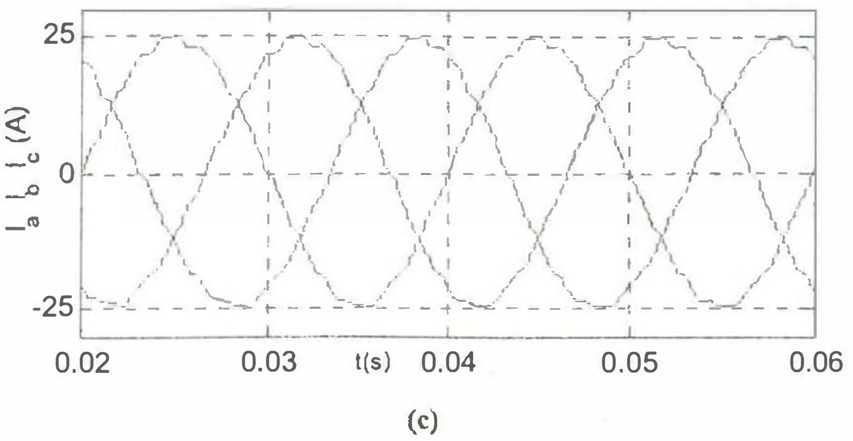
Şekil 12. L=80\text{mH} ve f_s=750\text{ Hz} için (a) Beş seviyeli faz gerilimi ve harmonik spektrumu (b) Dokuz seviyeli hat gerilimi ve harmonik spektrumu (c) Üç-faz akımları
