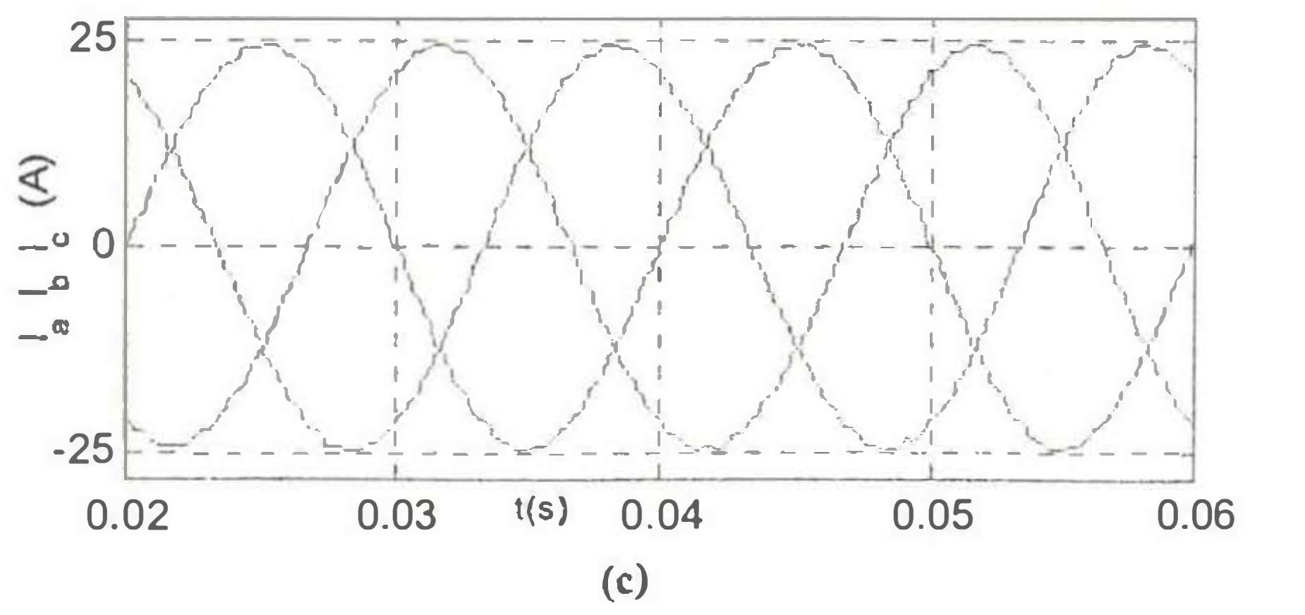
Şekil 13. L=80\text{mH} ve f_s=1250\text{ Hz} için (a) Beş seviyeli faz gerilimi ve harmonik spektrumu (b) Dokuz seviyeli hat gerilimi ve harmonik spektrumu (c) Üç-faz akımları
