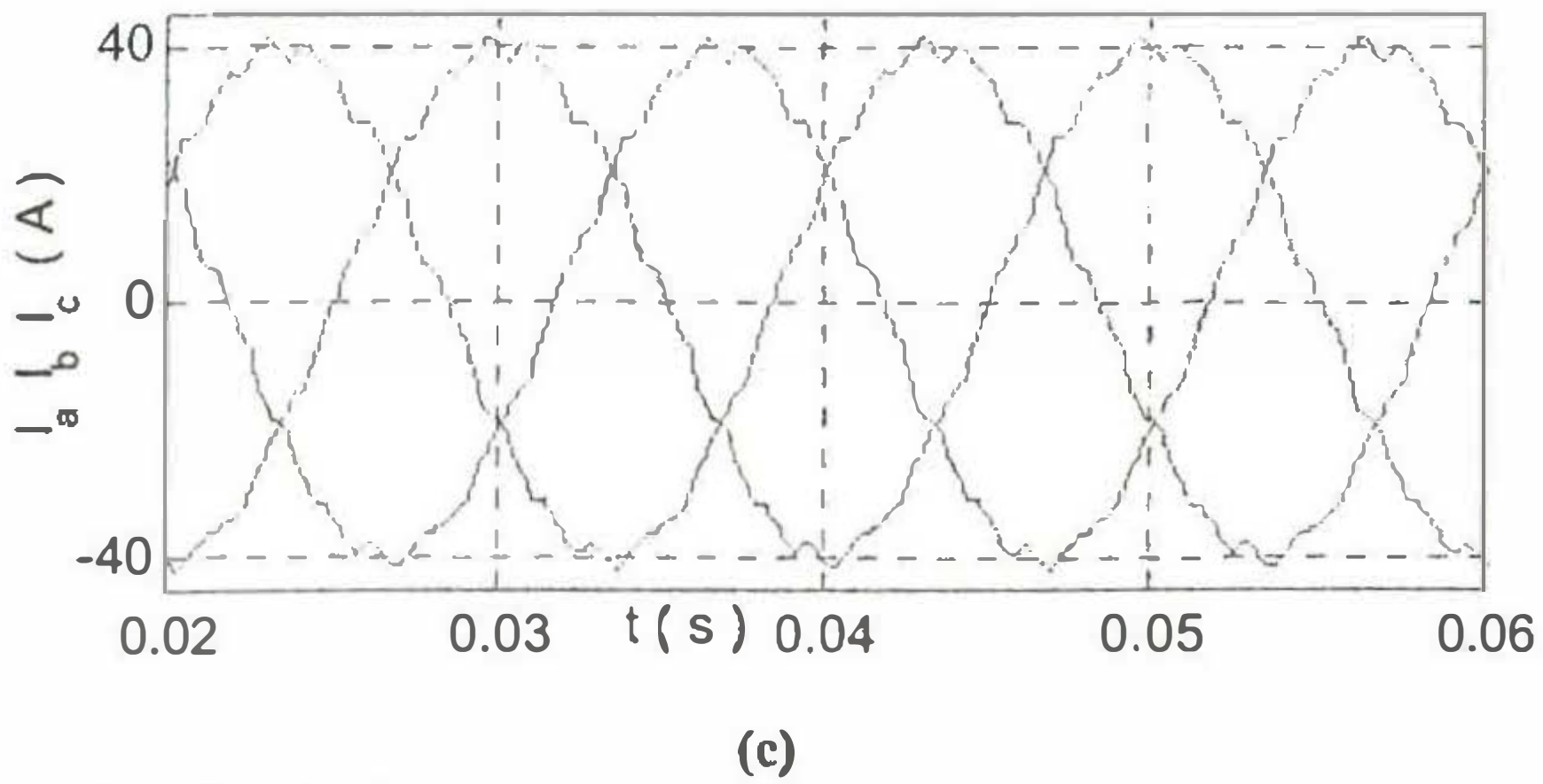
Şekil 10. L=30\text{mH} ve f_s=750\text{ Hz} için (a) Beş seviyeli faz gerilimi ve harmonik spektrumu (b) Dokuz seviyeli hat gerilimi ve harmonik spektrumu (c) Üç-faz akımları
