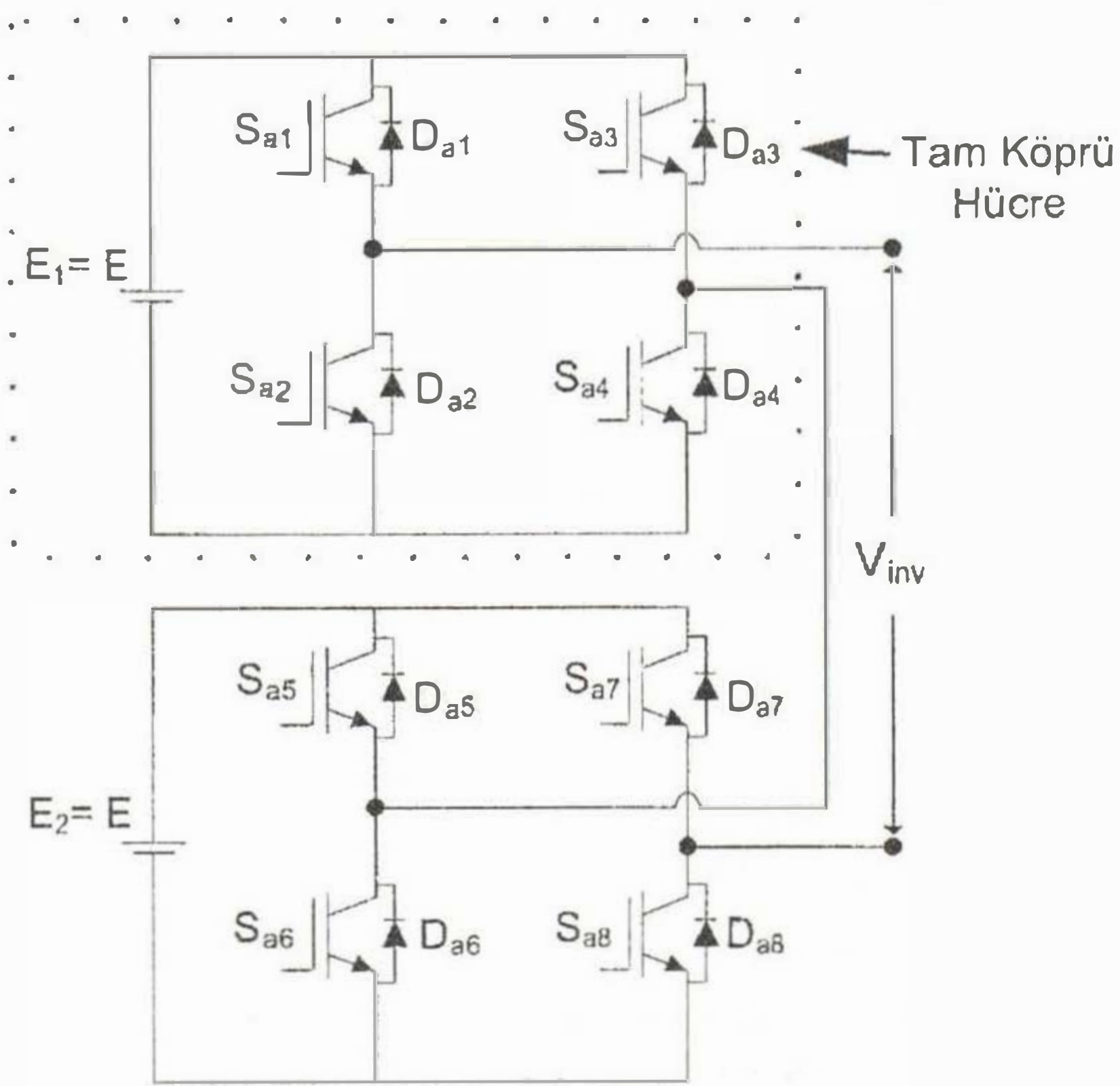
Şekil 2. Beş-seviyeli kaskat inverterin bir faz bacağı
