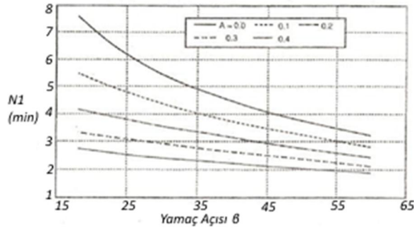
Şekil 9. Duraylılık sayısı N_1 'in ivme ve yamaç açısına göre değişimi (Number of stability, acceleration and slope angle change compared to N_1 )
