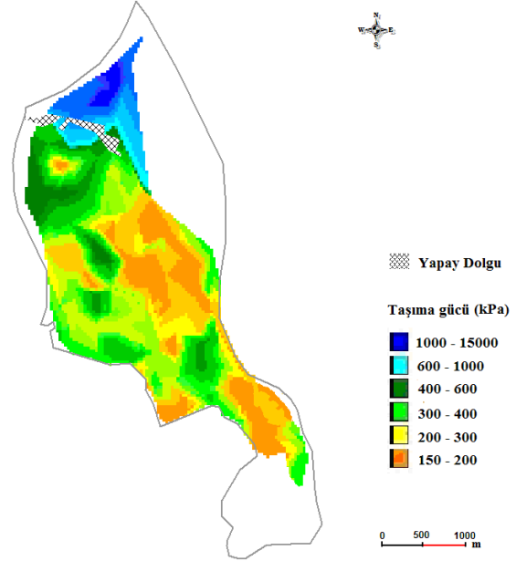
Şekil 11. İnceleme alanında yüzeyel temeller için hesaplanan güvenli taşıma güçleri ve kaya birimleri için hesaplanan izin verilebilir taşıma güçlerinin aynı haritada görünümü (The same view of the map can be calculated allowing for the safe carrying capacity carrying capacity and rocks in the study area are calculated for shallow foundations)
