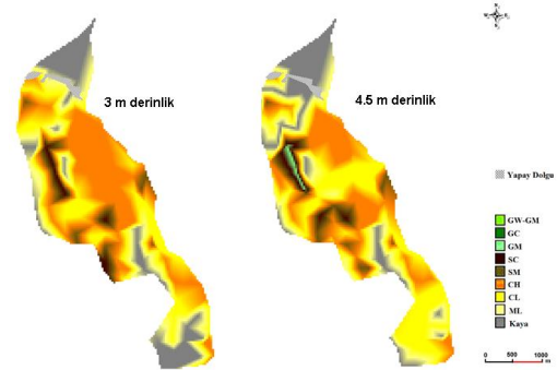
Şekil 6. Yüzeiden 3 m ve 4.5 m derinlikte zemin sınıflarının dağılım haritası (3 m and 4.5 m depth from the surface of the ground-class distribution map)
