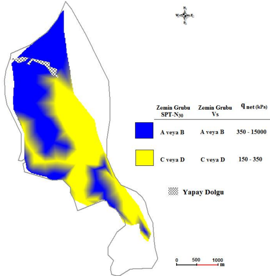
Şekil 13. Birinci grup sorgulamalara göre yerleşime uygunluk haritası (Settlement suitability map according to the first group inquiry)
