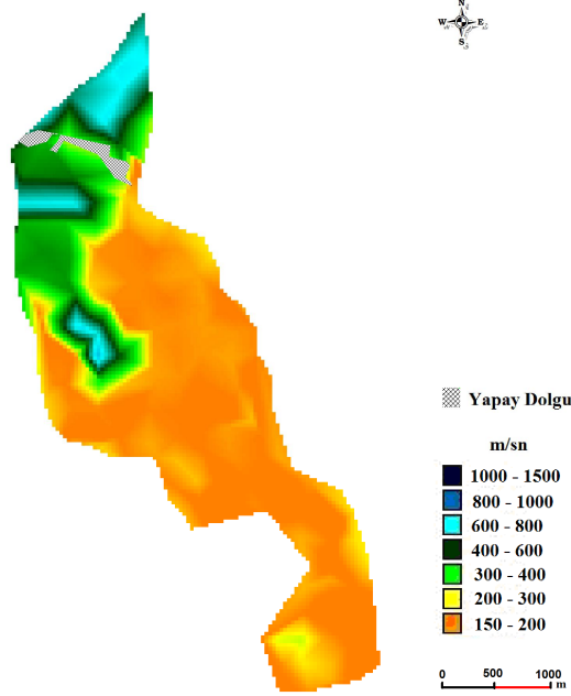
Şekil 5. Yüzeiden 5 m derinlikte kayma dalgası (Vs) hız dağılımı haritası (5 m depth from the surface shear wave (Vs) velocity distribution map)
