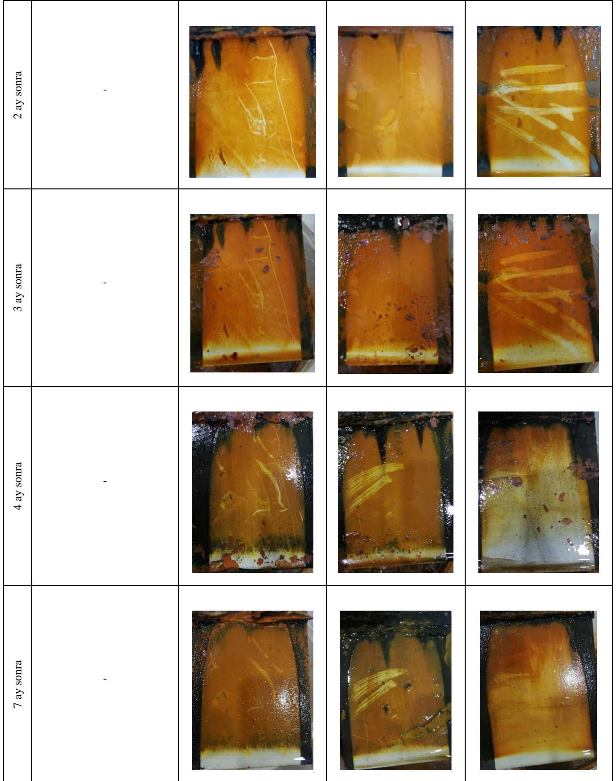
Şekil 6. Fenil floroborat katkılı boya ile muamele edilmiş metal levhaların deniz suyunda farklı sürelerde bekletildikten sonraki görüntüleri (Images of metal sheets treated with phenyl fluoroborate added paint after being kept in sea water for different periods)
