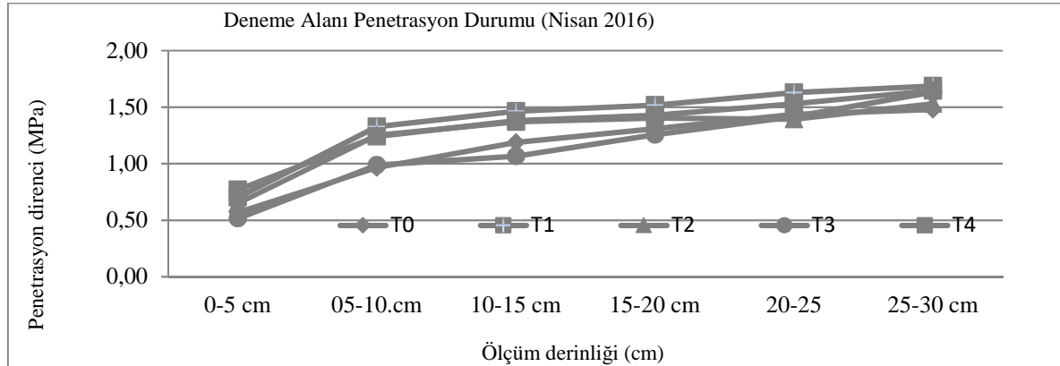
Şekil 5. Mısırın ekim öncesi farklı toprak derinliklerindeki penetrasyon direnci Figure 5. Penetration resistance of different depths of soil before sowing corn
