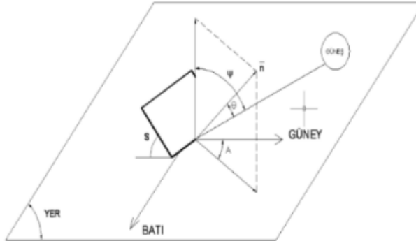
Şekil 8. Panellerin yerleştirilme açısı
