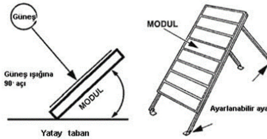
Şekil 3. Güneş panellerinin yerleştirildiği açı
