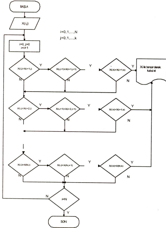
Şekil 2: Referans Tablonun Verilen Toleransla Azaltımı.
