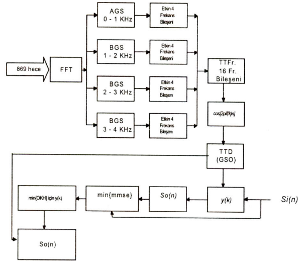
Şekil 1: Temel Tanım Dizileri ile Konuşma İşaretinin Modellenmesi.
