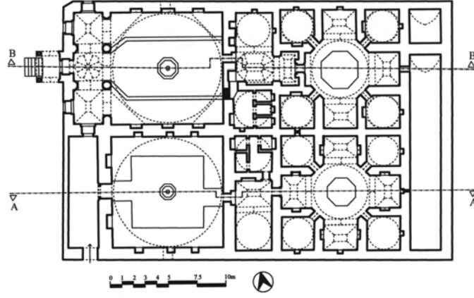
Çizim 3: Yeni Hamam Planı
