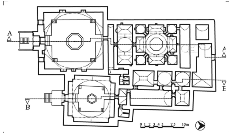
Çizim 1: Eski Hamam Planı (V.G.M. Arşivi'nden düzeltilerek).
