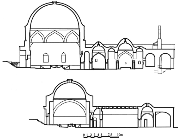
Çizim 2: Eski Hamam A-A ve B-B kesiti (V.G.M. Arşivi'nden düzeltilerek).
