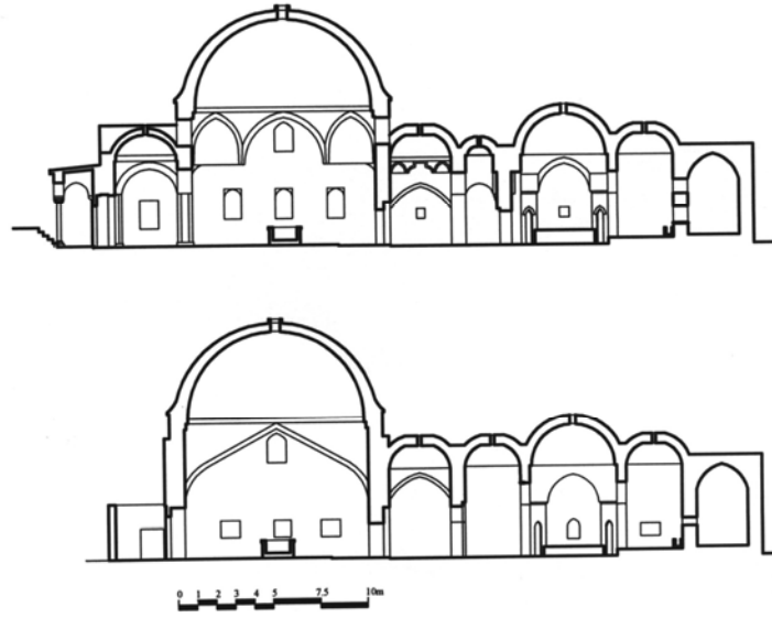
Çizim 4: Yeni Hamam A-A ve B-B Kesiti
