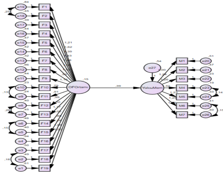
Şekil 1. Modelin AMOS Diyagramı
