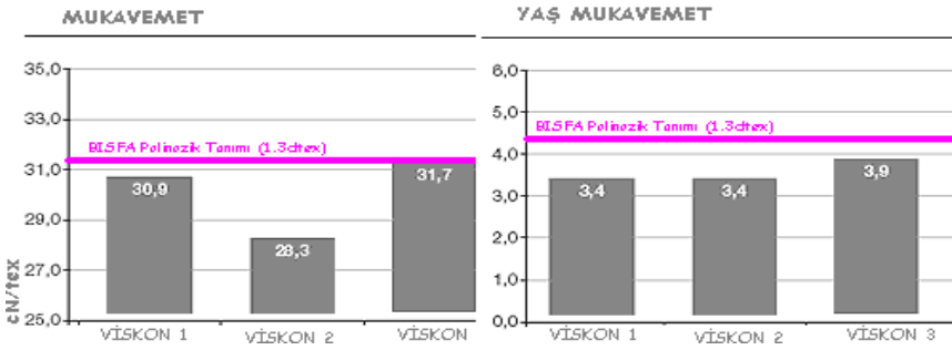
Şekil 12. Polinozik Liflerin Kuru ve Yaş Mukavemetleri (14)
