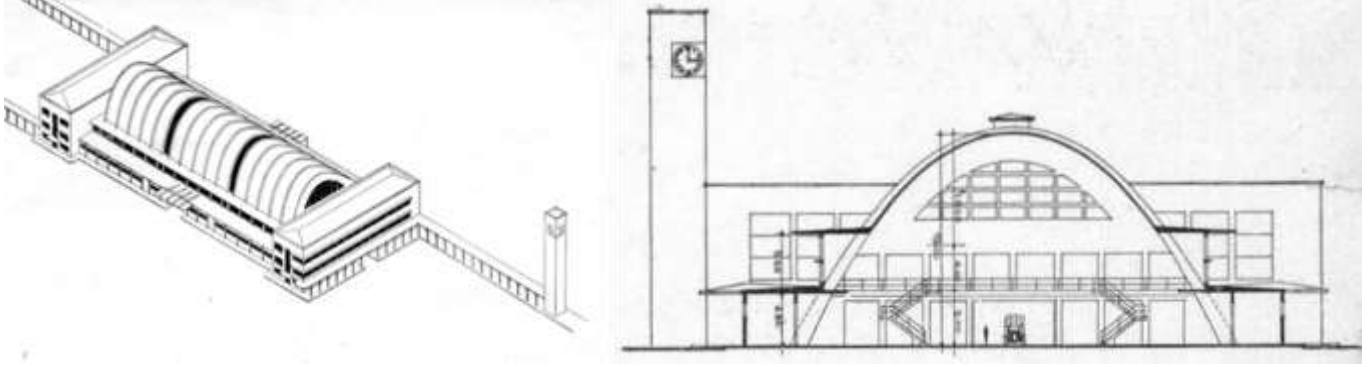
Resim 4., 5. İzmir Hal Santrali yarışmasını kazanan projenin perspektif ve ön cephesi (Arkitekt, 1937,b)
