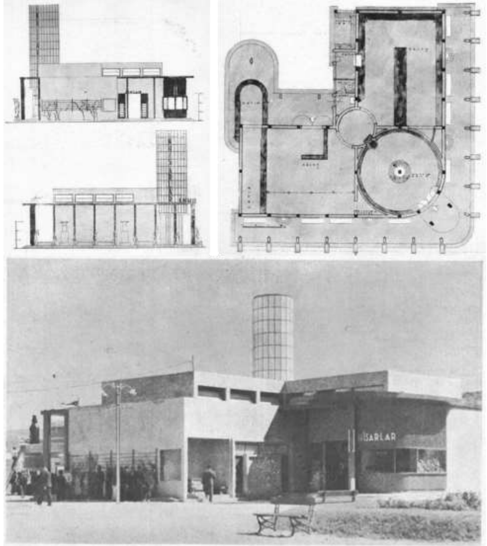
Resim 1., 2., 3. ‘İzmir Fuarı İnhisarlar Pavyonu’ yarışmasını kazanan projenin cephe ve plan çizimleri, projenin uygulanmış hali (Uzman, 1936)
